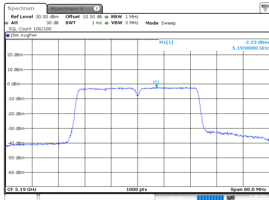
n40_5190MHz
