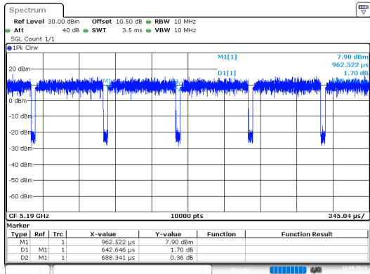
n40_5190MHz
