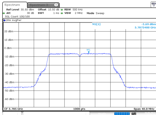
a_5785MHz
