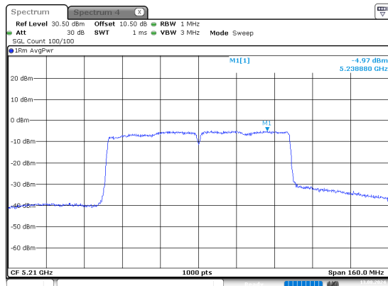
ac80_5210MHz
