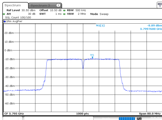
n40_5795MHz
