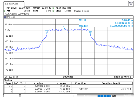
a_5200MHz
