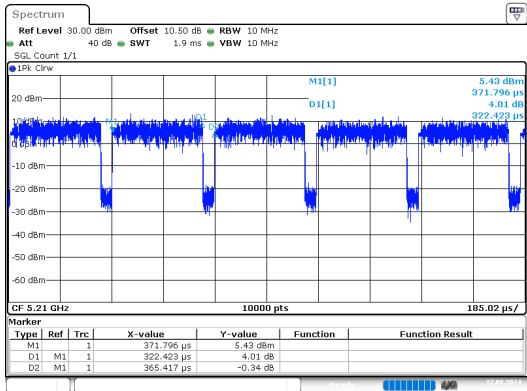
ac80_5210MHz
