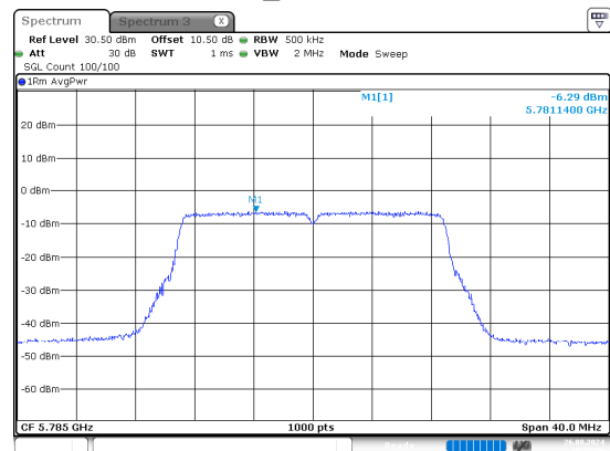
n20_5785MHz
