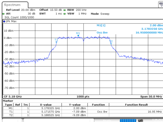
a_5180MHz
