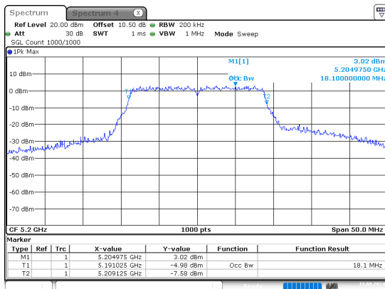
n20_5200MHz
