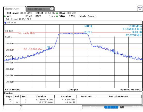
n20_5180MHz
