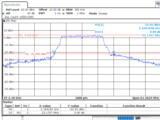
a_5180MHz
