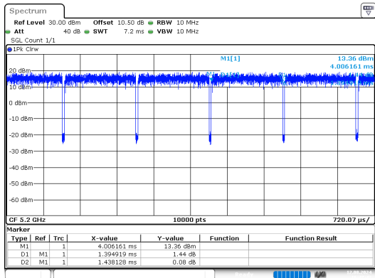
a_5200MHz
