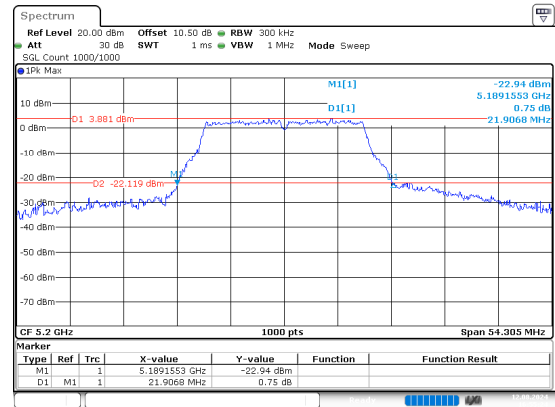
a_5200MHz
