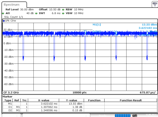
n20_5200MHz
