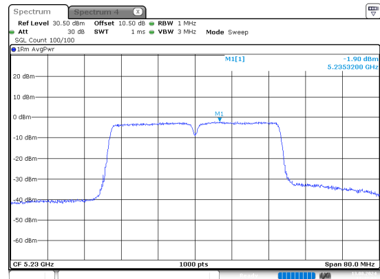
n40_5230MHz
