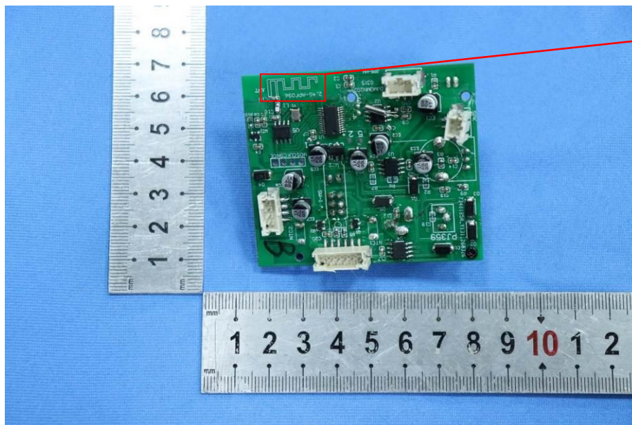
2.4G antenna
