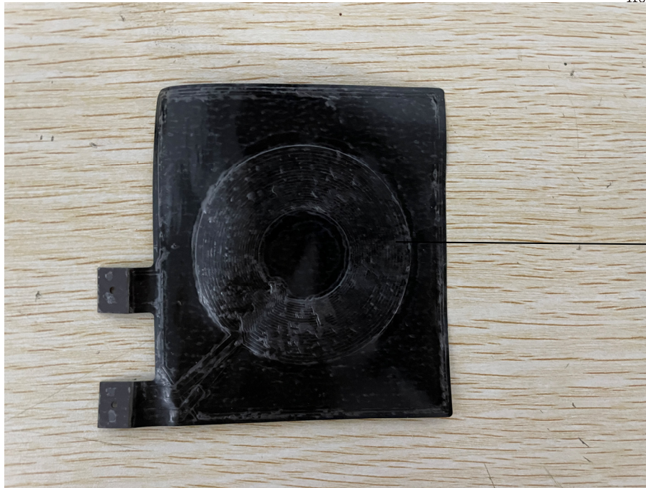
WPC/NFC Antenna
