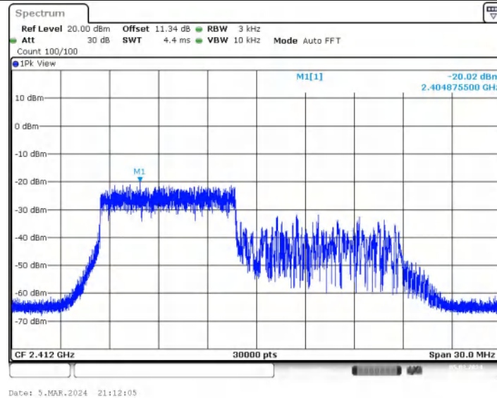
11AX20MIMO_Ant2_2412_106Tone_RU54
