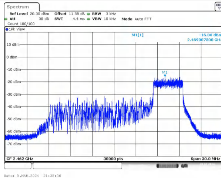
11AX20MIMO_Ant2_2462_106Tone_RU53
