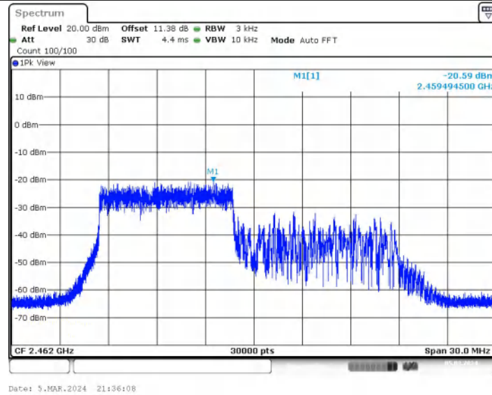
11AX20MIMO_Ant2_2462_106Tone_RU54
