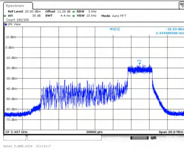
11AX20MIMO_Ant1_2437_106Tone_RU53
