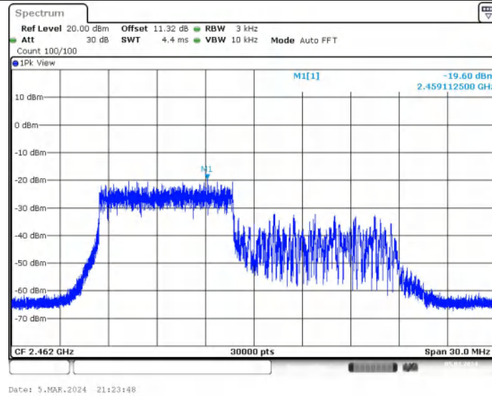
11AX20MIMO_Ant1_2462_106Tone_RU54
