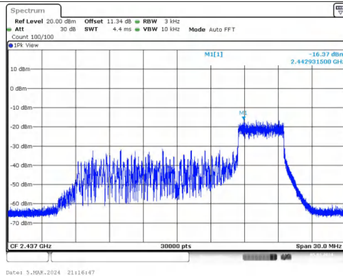
11AX20MIMO_Ant2_2437_106Tone_RU53
