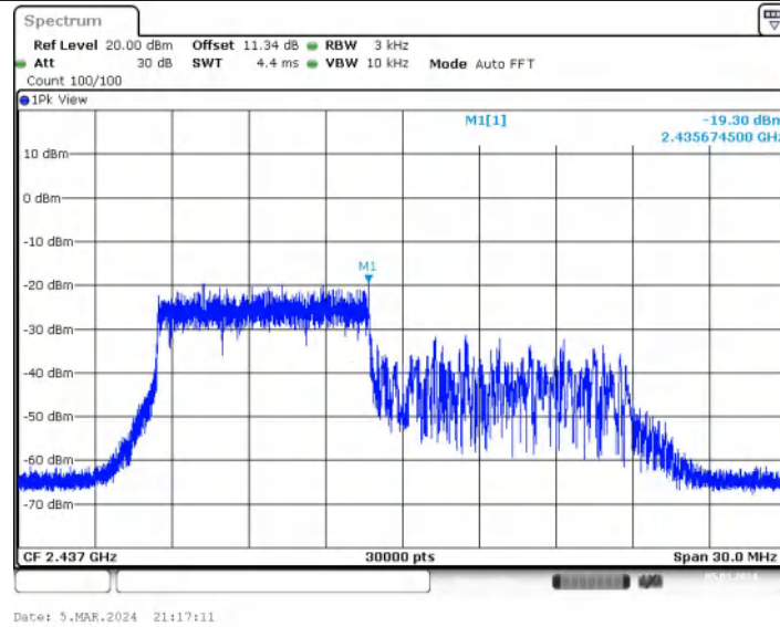
11AX20MIMO_Ant2_2437_106Tone_RU54
