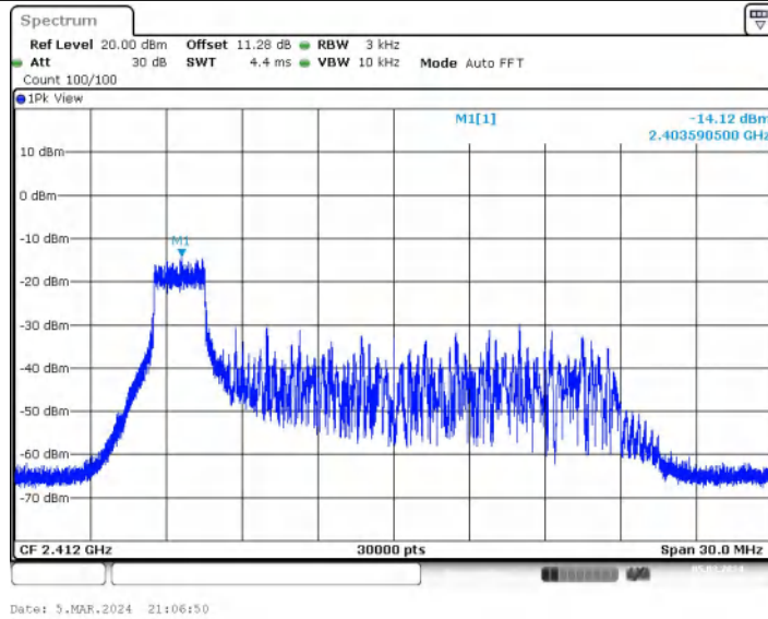
11AX20MIMO_Ant1_2412_26Tone_RU8
