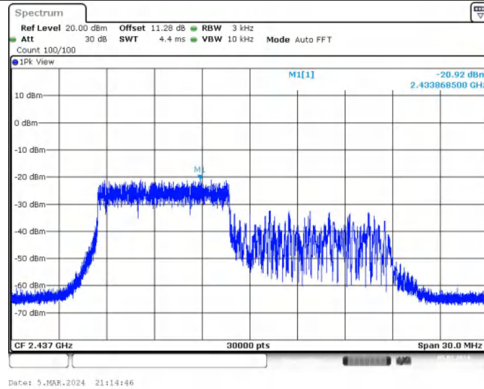
11AX20MIMO_Ant1_2437_106Tone_RU54
