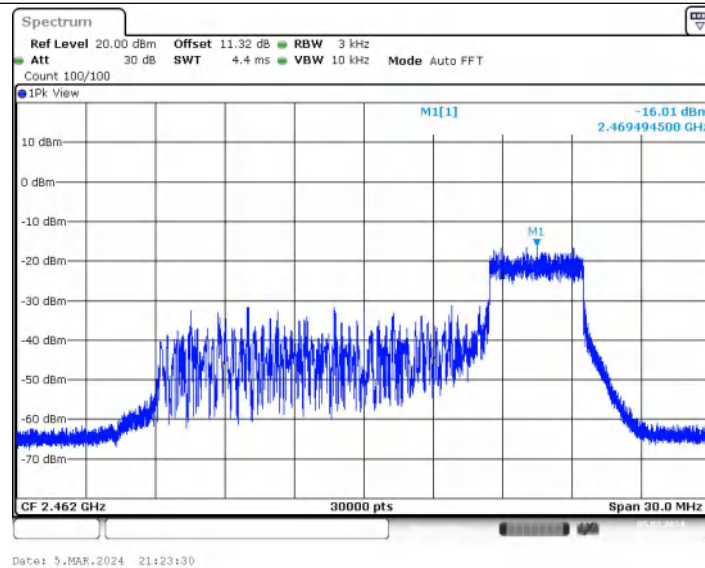
11AX20MIMO_Ant1_2462_106Tone_RU53
