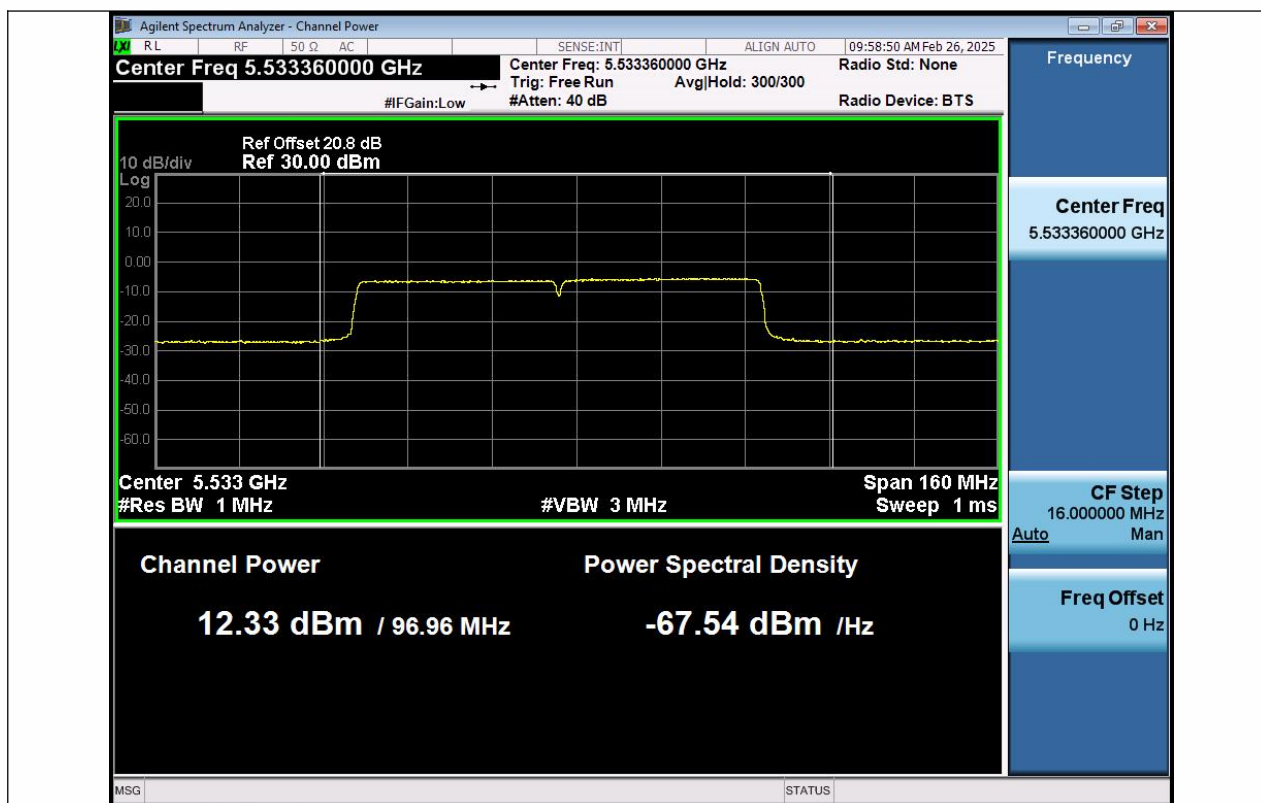
11AC80SISO-Ant1-5530-PASS
