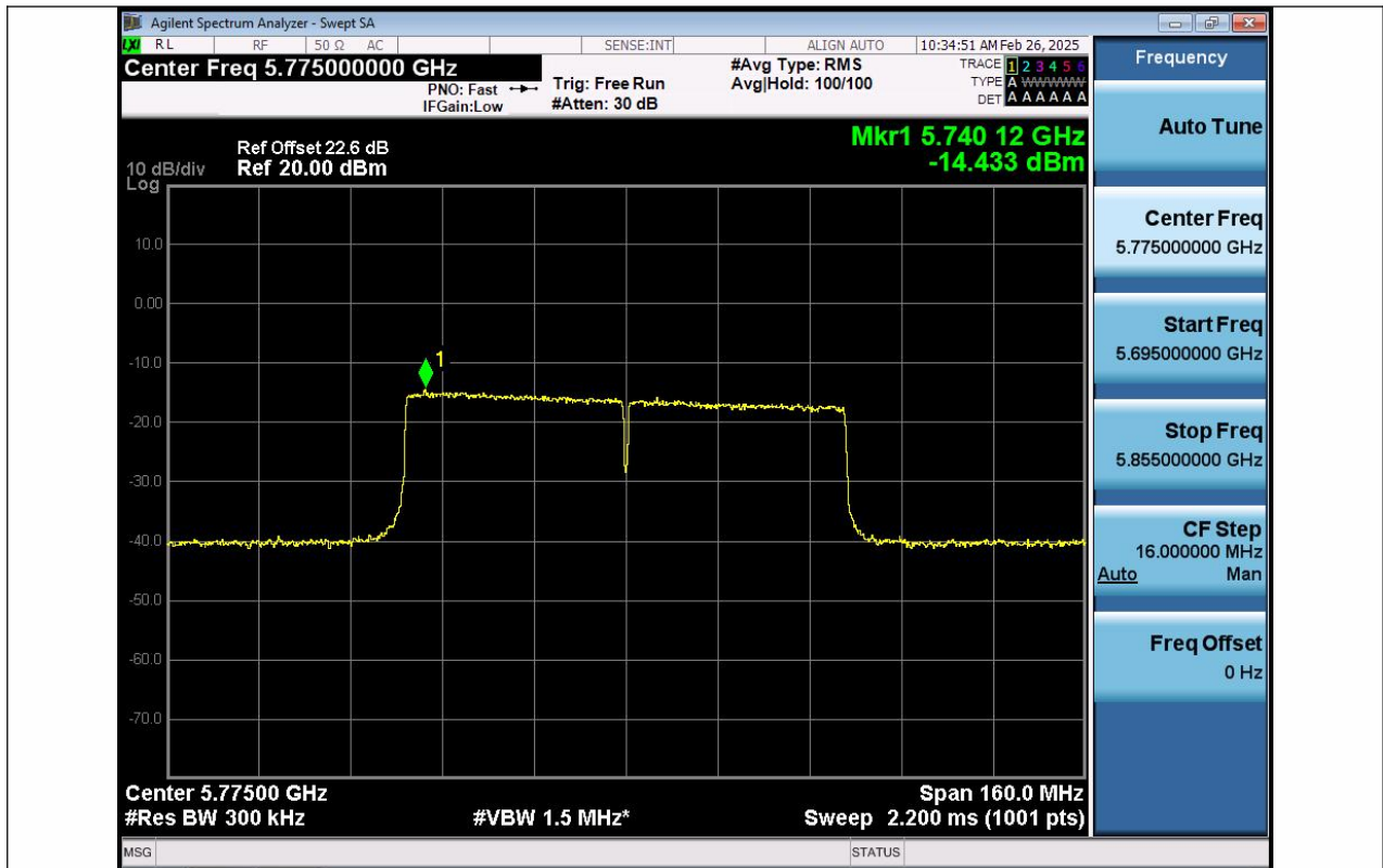
11AC80SISO-Ant1-5775-PASS
