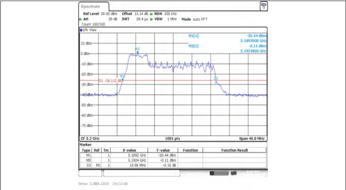
11AX20MIMO-Ant1-5200-52Tone-RU37
