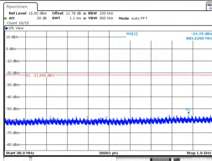
11AX20MIMO_Ant1_2412_26Tone_RU0_30~1000
