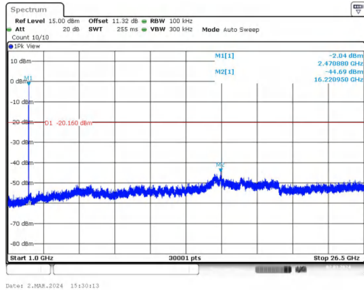
11AX20MIMO_Ant1_2462_52Tone_RU37_0~Reference
