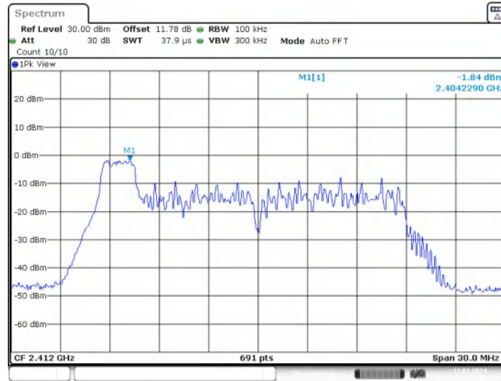
11AX20MIMO_Ant1_2412_26Tone_RU0_0~Reference
