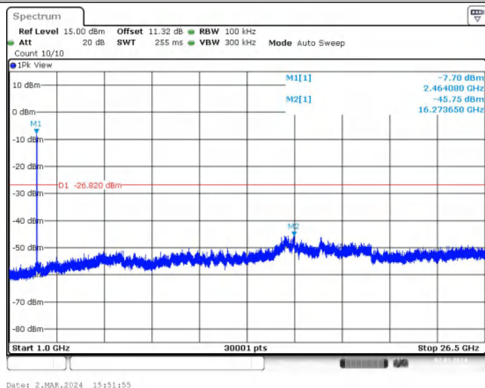
11AX20MIMO_Ant1_2462_106Tone_RU54_1000~26500
