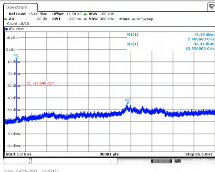
11AX20MIMO_Ant1_2412_106Tone_RU53_1000~26500
