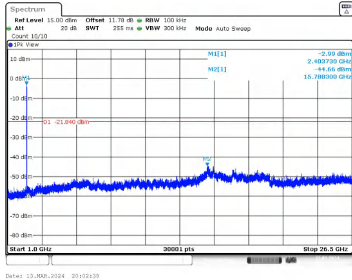
11AX20MIMO_Ant1_2412_26Tone_RU8_0~Reference
