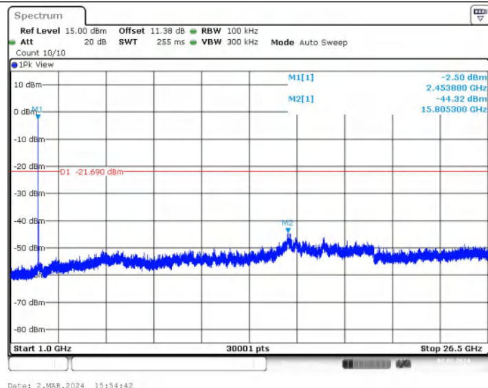
11AX20MIMO_Ant2_2462_26Tone_RU8_0~Reference
