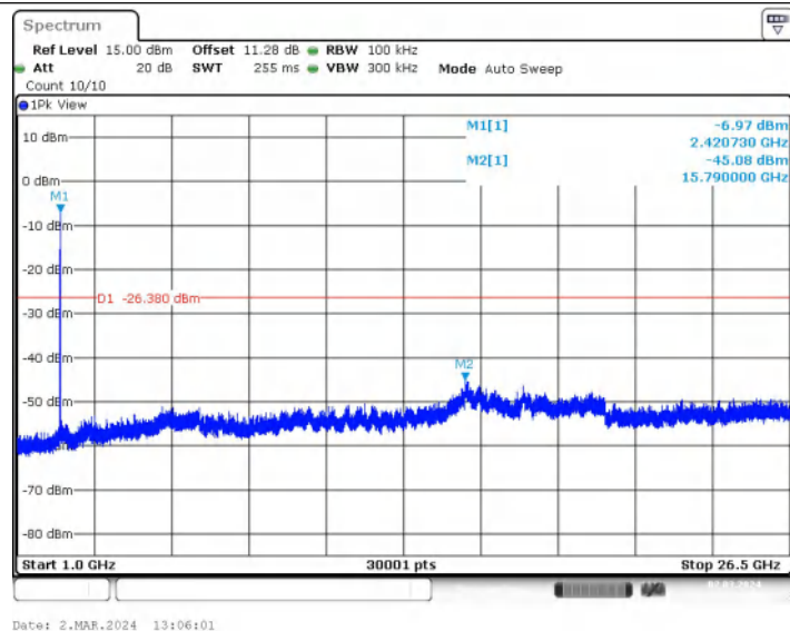
11AX20MIMO_Ant2_2412_26Tone_RU0_0~Reference
