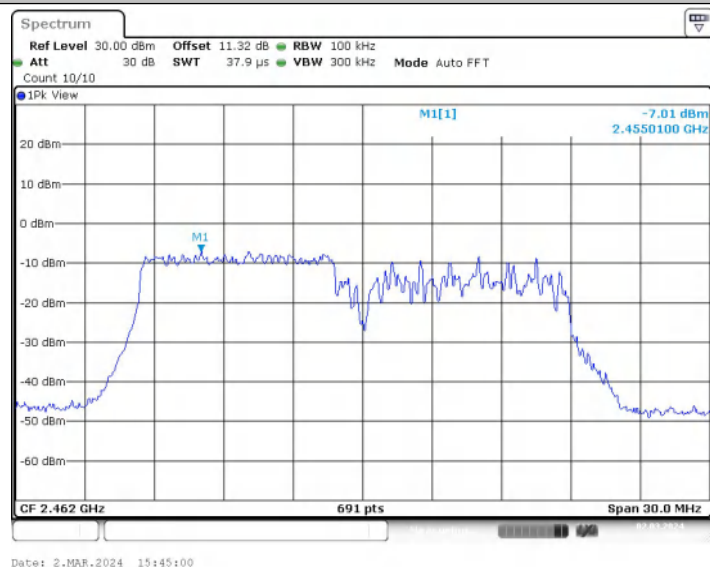
11AX20MIMO_Ant1_2462_106Tone_RU53_0~Reference
