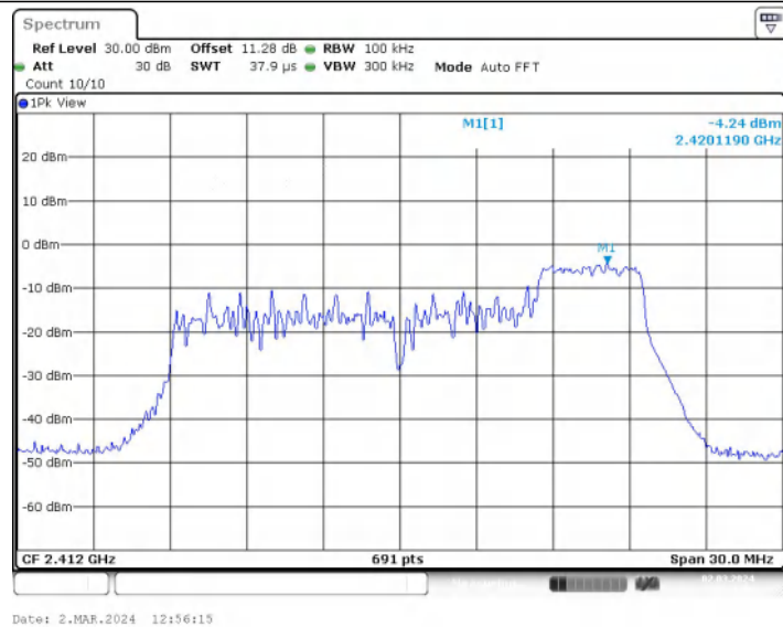
11AX20MIMO_Ant1_2412_52Tone_RU40_0~Reference
