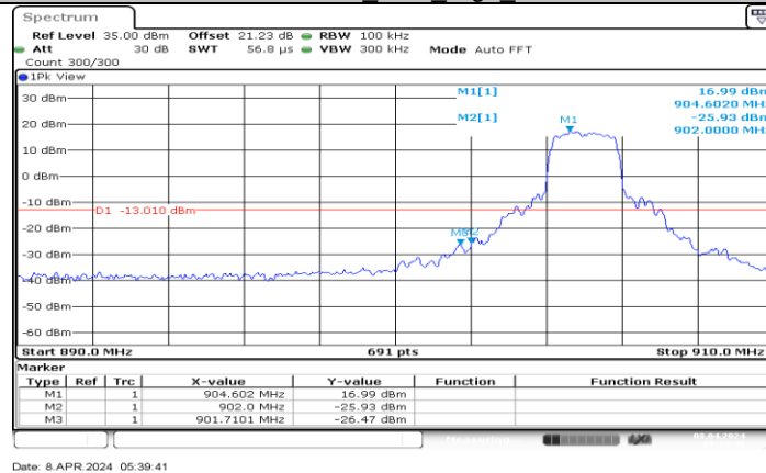
802.11ah 2M_Ant1_Low_905
