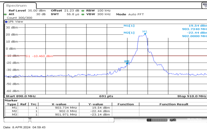
802.11ah 1M_Ant1_Low_903.5
