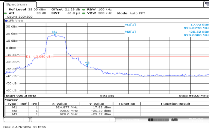
802.11ah 2M Ant1 High 925
