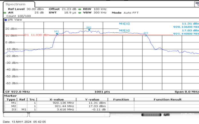
802.11ah 4M Ant1 922
