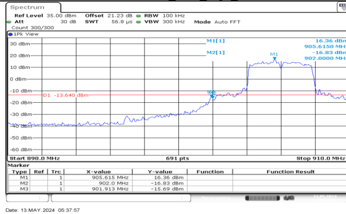
802.11ah 4M Ant1 Low 906
