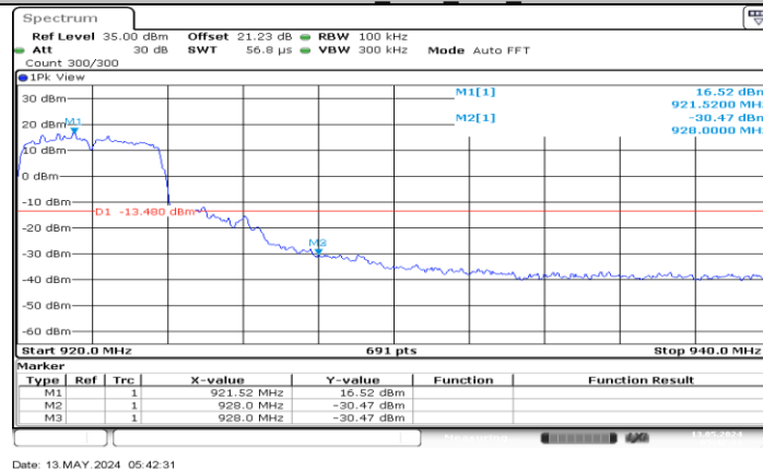
802.11ah 4M Ant1 High 922
