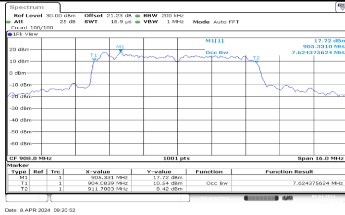
802.11ah 8M Ant1_908
