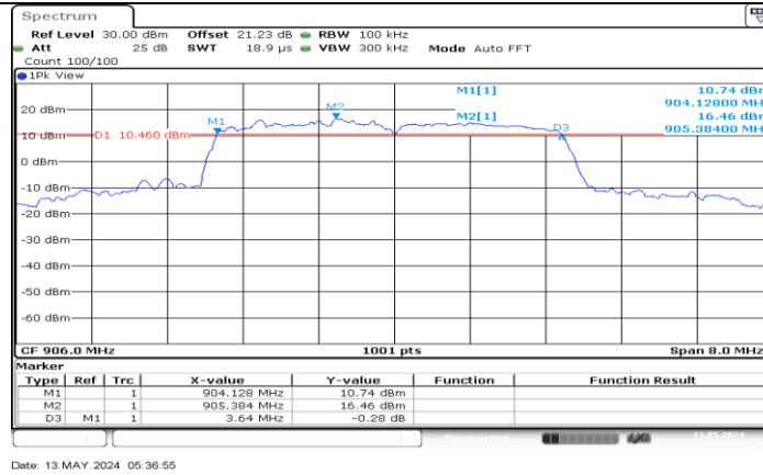
802.11ah 4M Ant1 906
