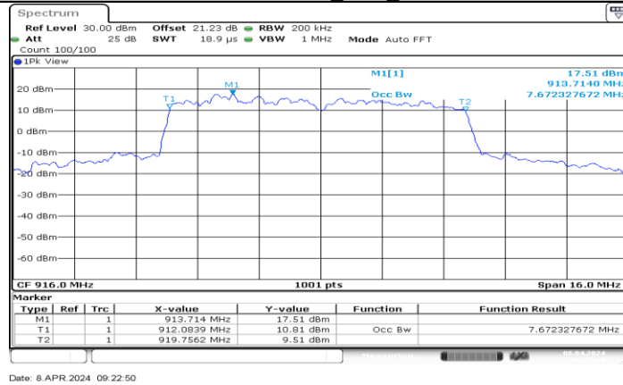
802.11ah 8M Ant1_916
