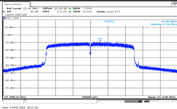
802.11ah 8M_Ant1_908
