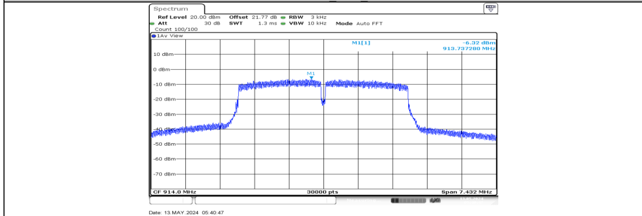
802.11ah 4M Ant1 914
