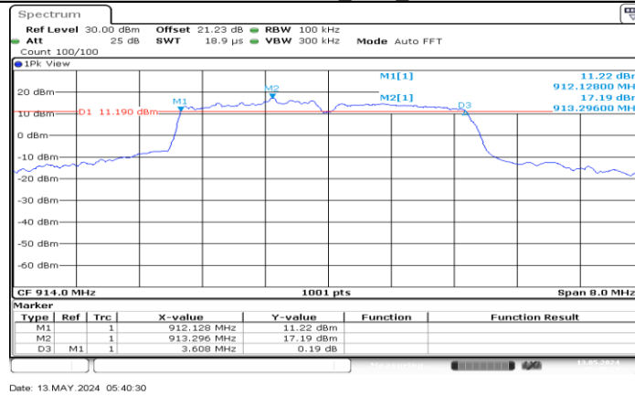
802.11ah 4M Ant1 914
