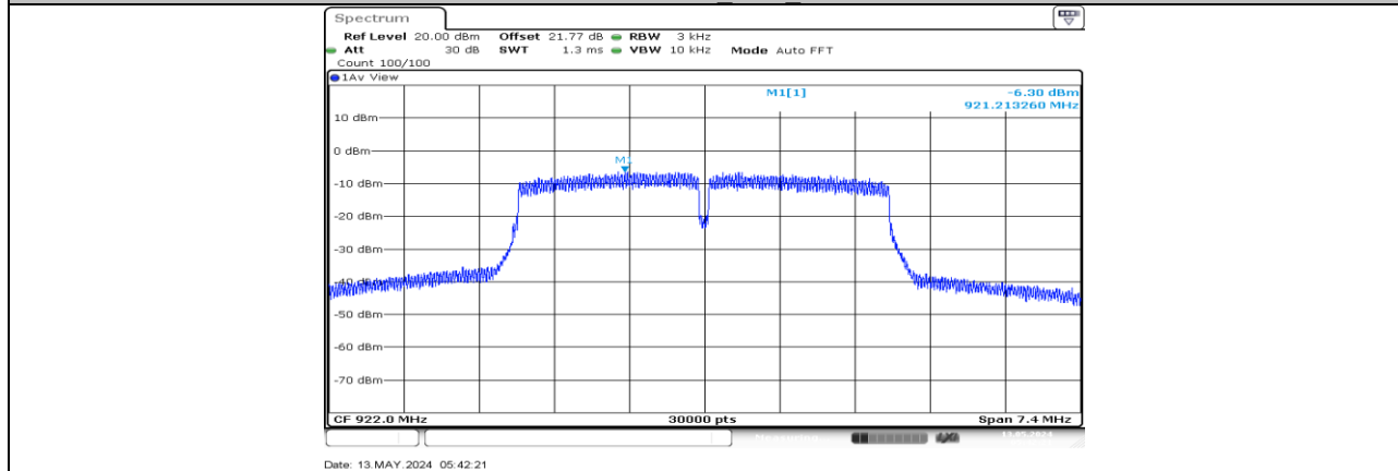
802.11ah 4M Ant1 922
