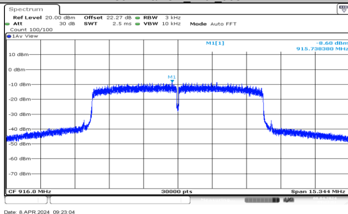
802.11ah 8M_Ant1_916
