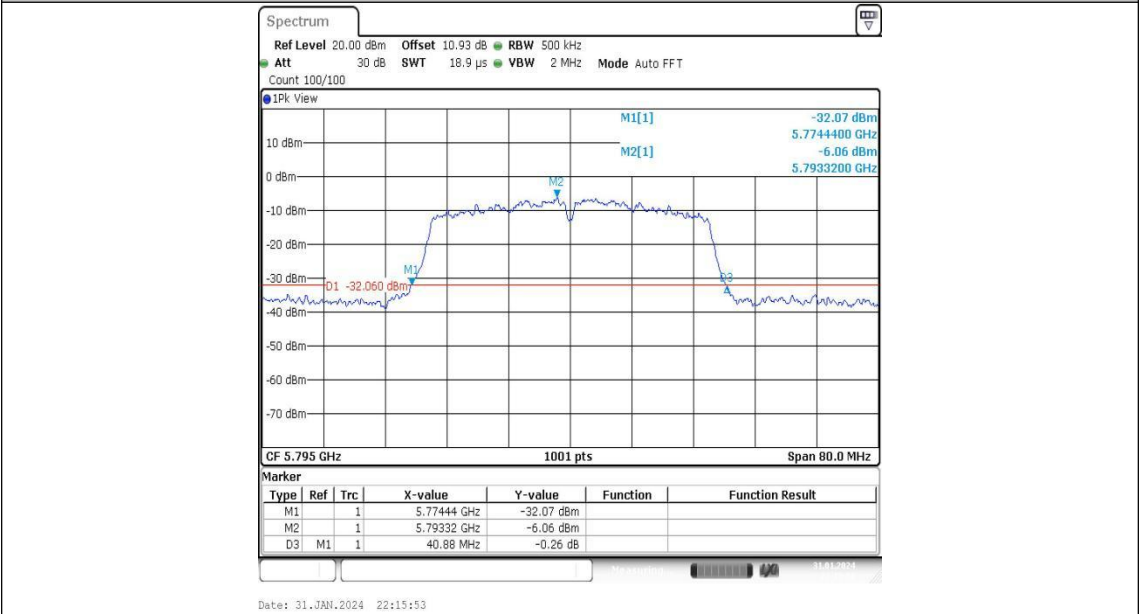
11N40MIMO-Ant2-5795
