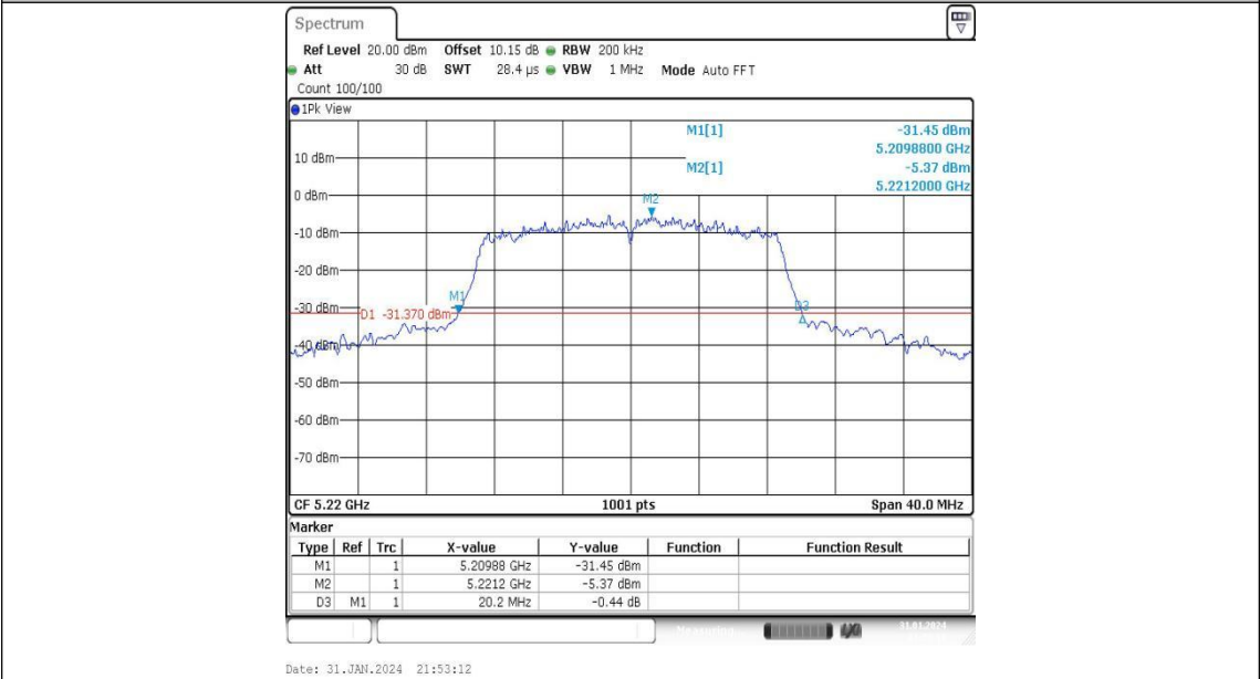
11N20MIMO-Ant2-5220
