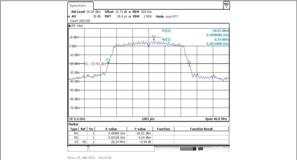
11N20MIMO-Ant1-5500
