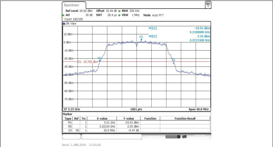
11A-Ant1-5220
