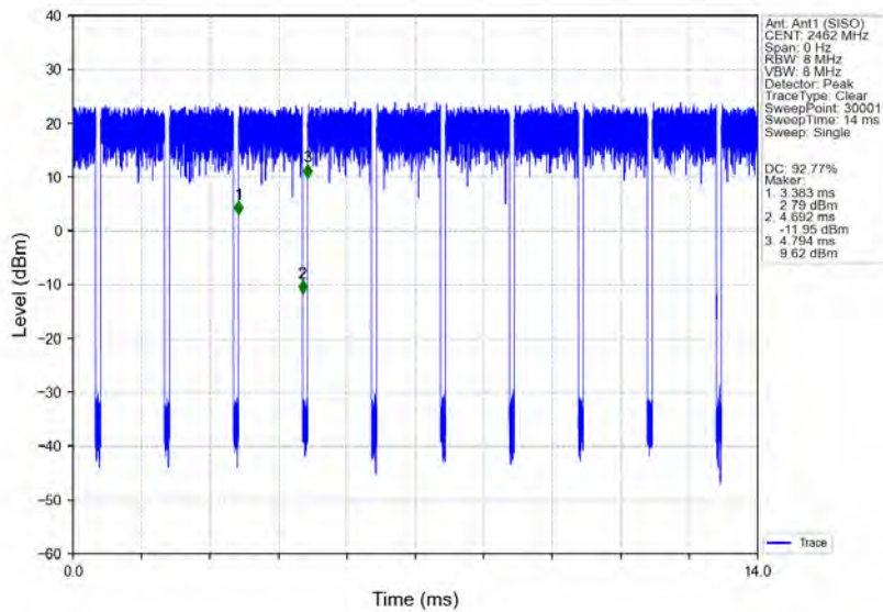
802.11n(HT20) HCH 2462MHz Ant1 (SISO) NTVN
