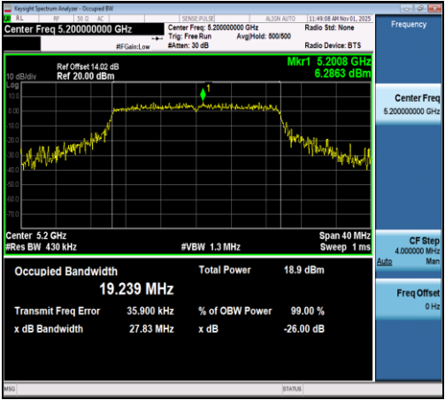
11AX20SISO-Ant1-5200
