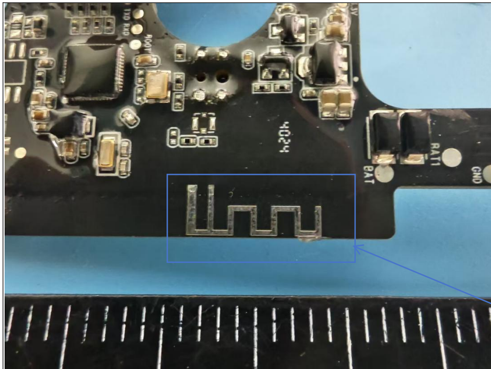
BLE ANTENNA
