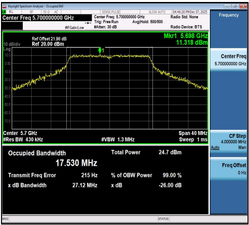
11A-Ant1-5700
