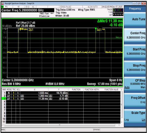
NTNV-11A-Ant1-5280
