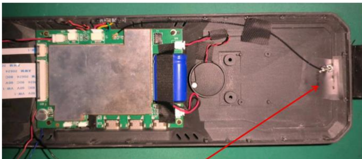
WIFI&BT天线 位置示意图
