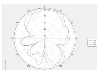
Phi 90 2D 图
