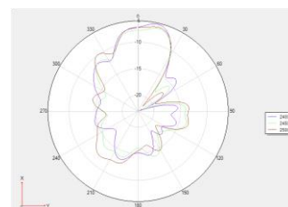
Theta 90 2D 图
