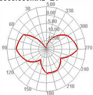
5500.000MHz E1
