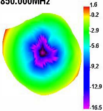
5850.000MHz
