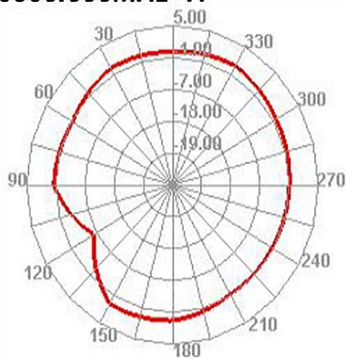
5850.000MHz H
