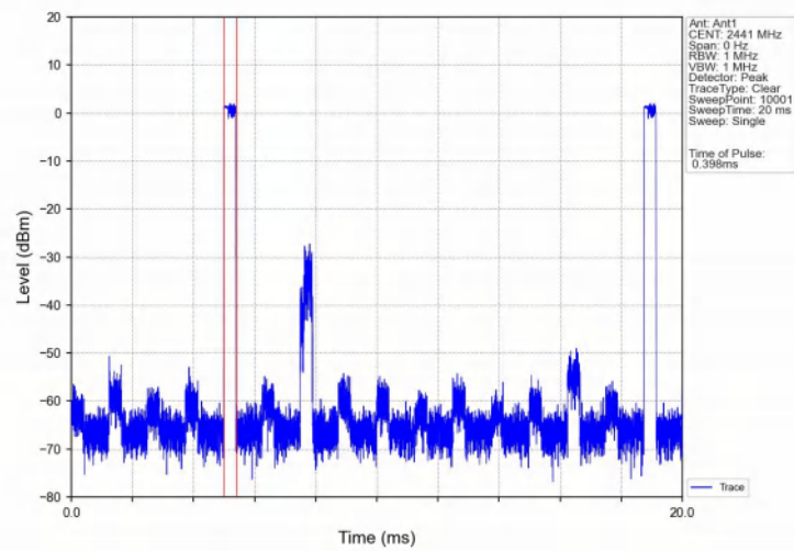
8DPSK_3DH1_HOPP_Ant1_NTNV
