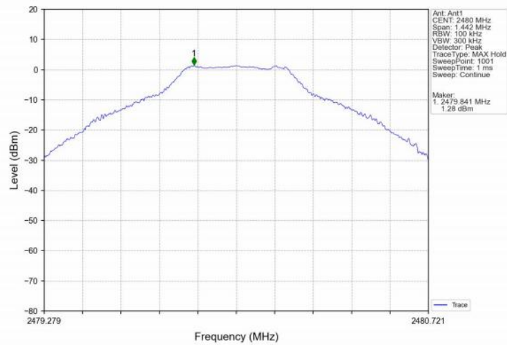
GFSK_DH5_HOPP_2480MHz_Ant1_NTNV
