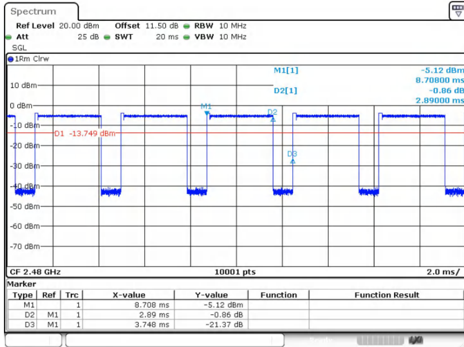
\pi/4 DQPSK(2-DH5)_Channel 78
