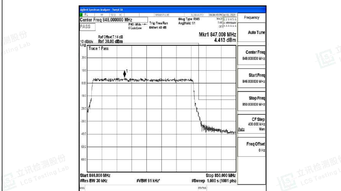
Band5_3MHz_QPSK_20635_15RB#0
