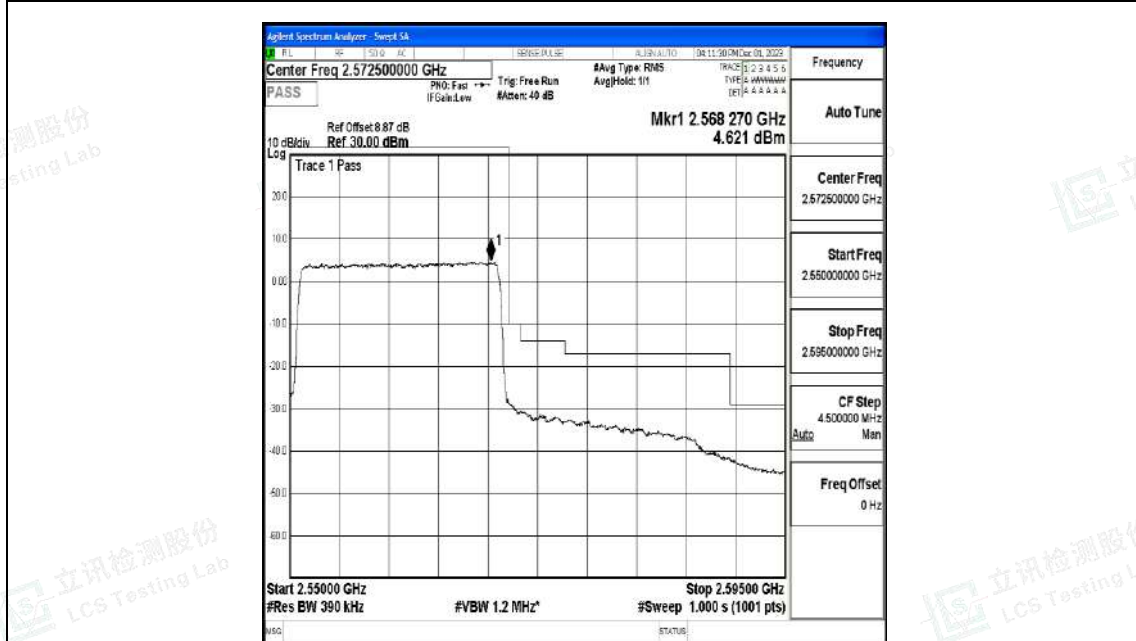
Band7_20MHz_16QAM_21350_100RB#0
