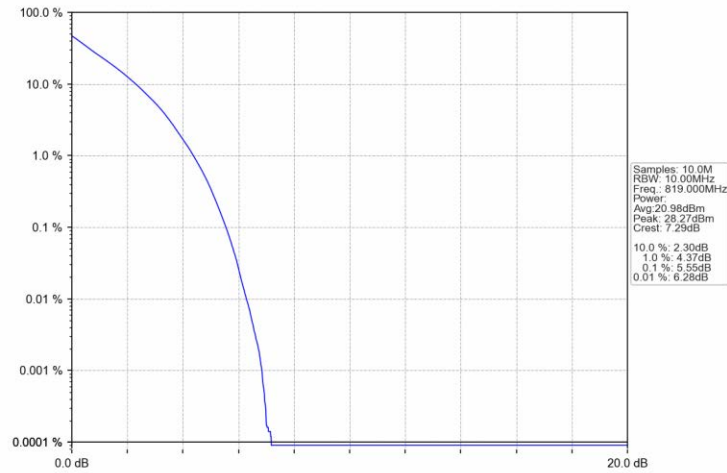
Band26a 10MHz QPSK MCH 819MHz RB 50 0 NTV
