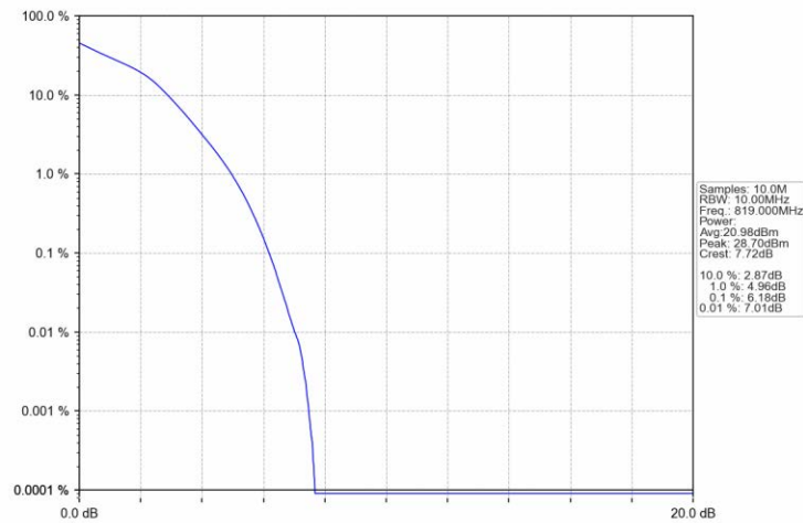
Band26a 10MHz 16QAM MCH 819MHz RB 50 0 NTV
