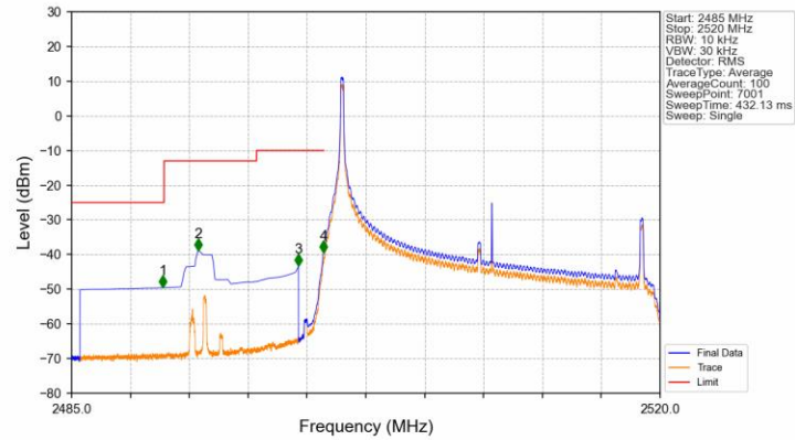
Band7 20MHz QPSK LCH 2510MHz RB 1 0 NTN
