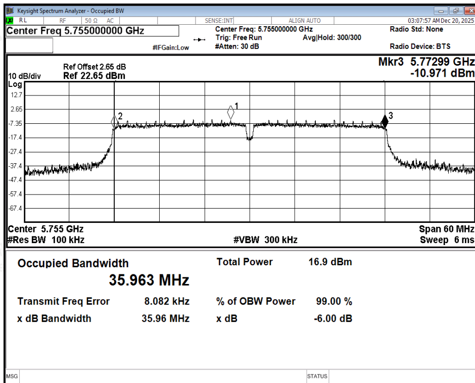
-6dB Bandwidth NVNT ax40 5755MHz Ant1
