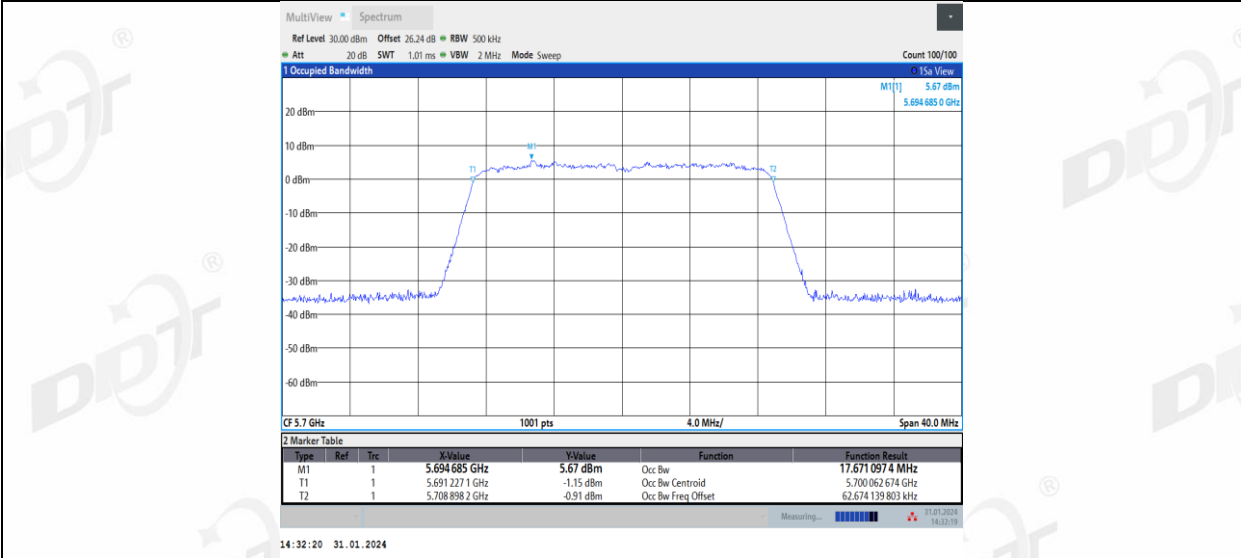
11AC20MIMO_Ant2_5700
