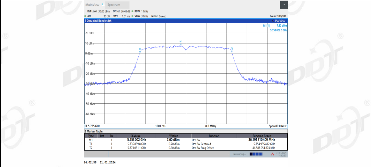
11N40MIMO_Ant2_5755
