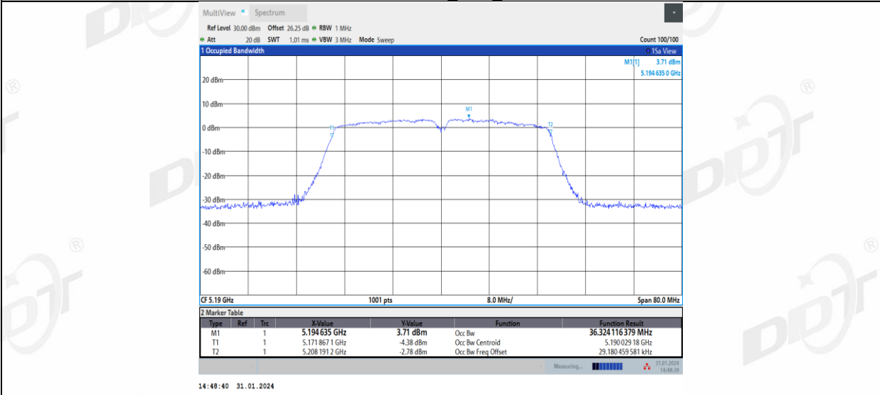
11AC40MIMO_Ant2_5190
