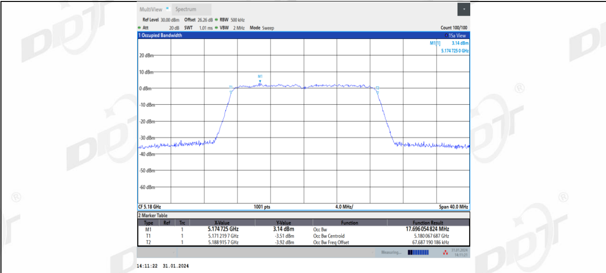
11AC20MIMO_Ant2_5180
