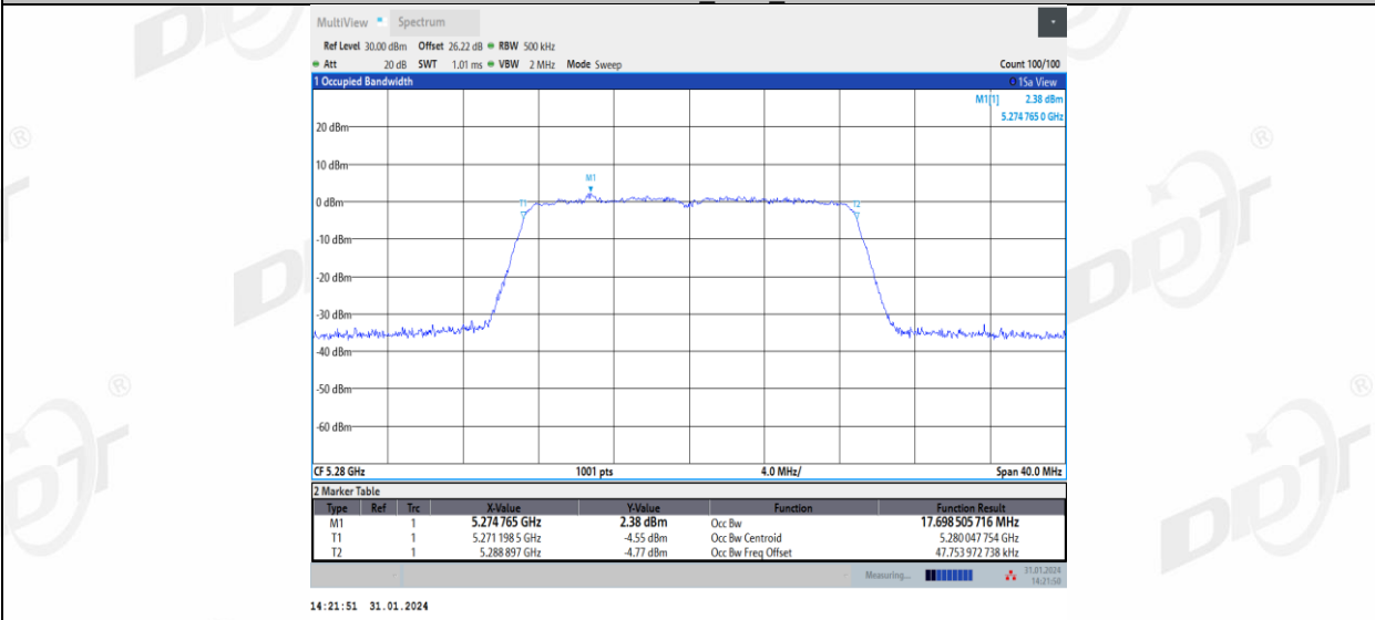
11AC20MIMO_Ant2_5280
