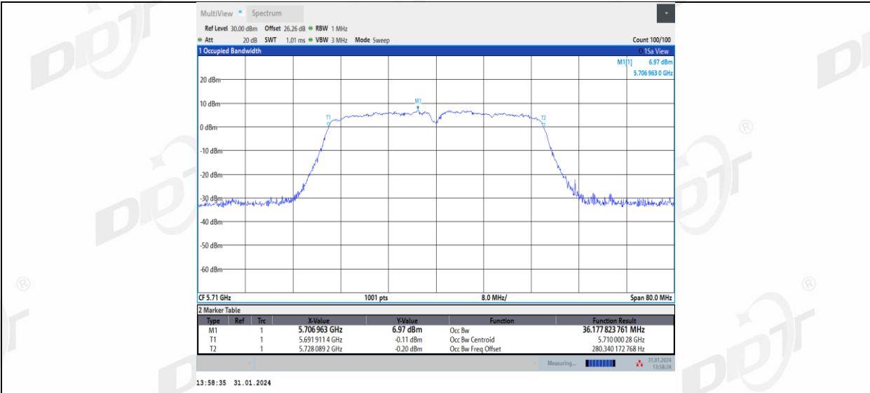
11N40MIMO_Ant2_5710
