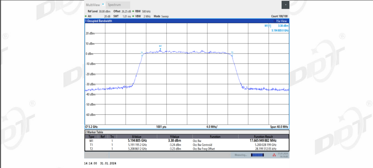
11AC20MIMO_Ant2_5200
