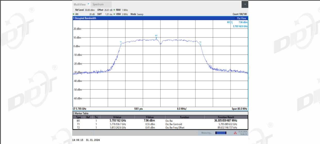
11N40MIMO_Ant2_5795
