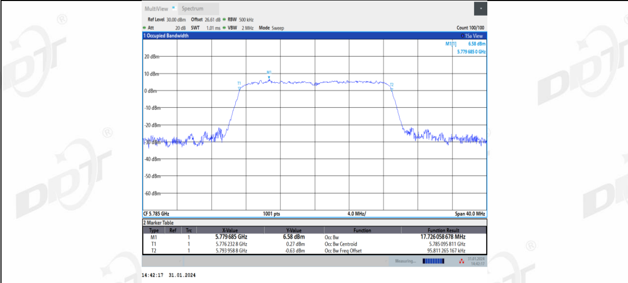
11AC20MIMO_Ant2_5785
