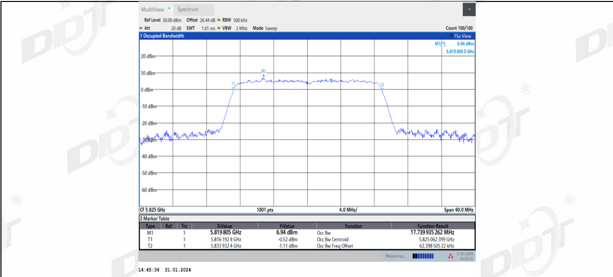
11AC20MIMO_Ant2_5825
