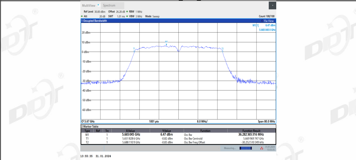
11N40MIMO_Ant2_5670
