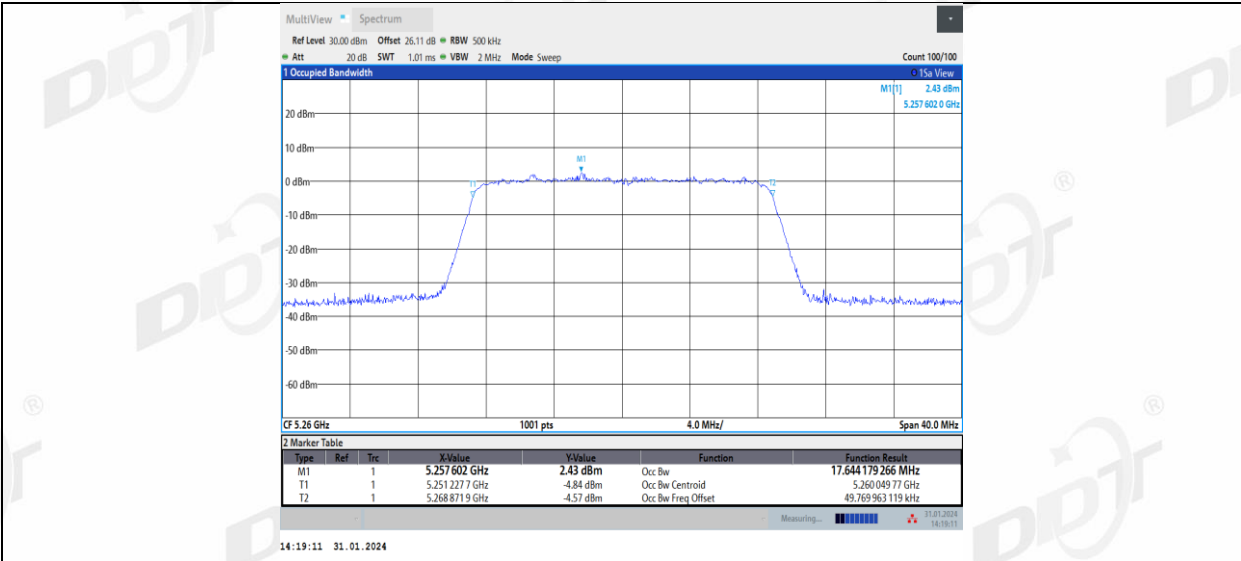
11AC20MIMO_Ant2_5260
