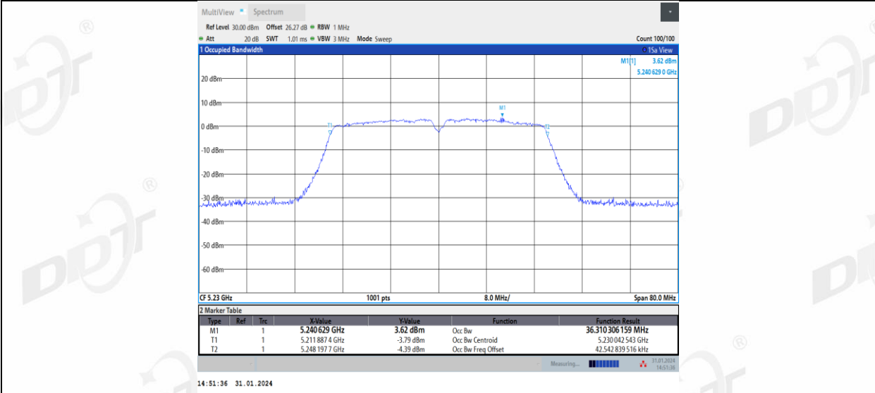
11AC40MIMO_Ant2_5230
