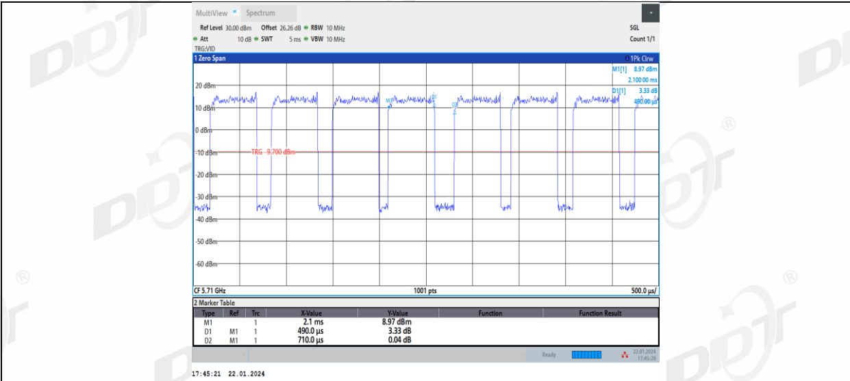
11N40MIMO_Ant2_5710
