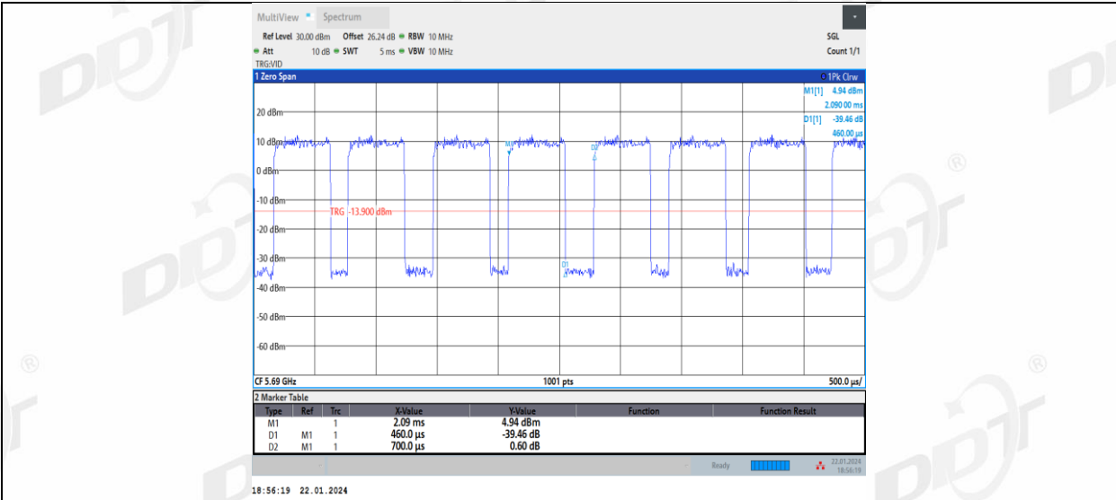
11AC80MIMO_Ant2_5690
