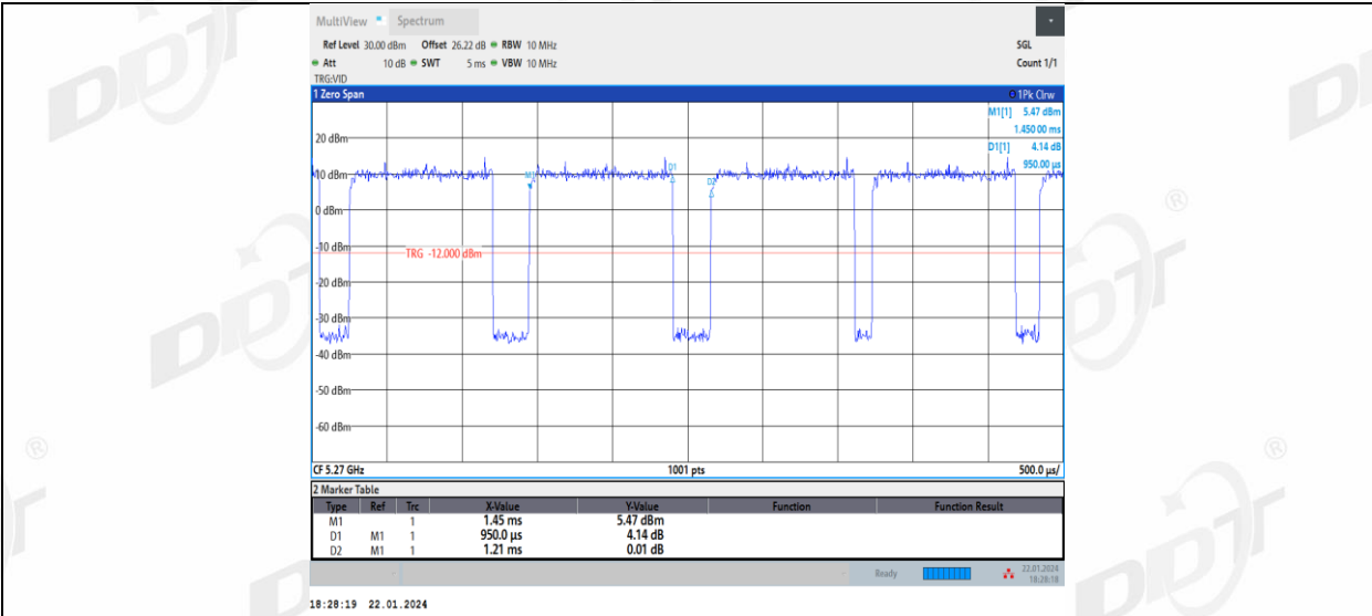
11AC40MIMO_Ant2_5270
