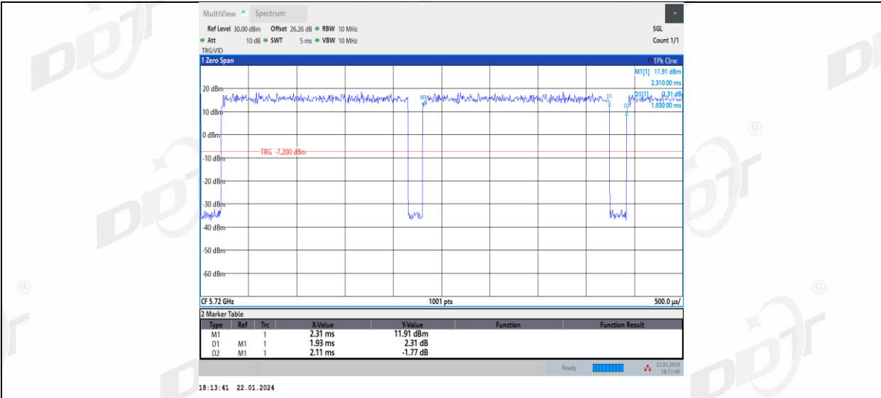
11AC20MIMO_Ant2_5720
