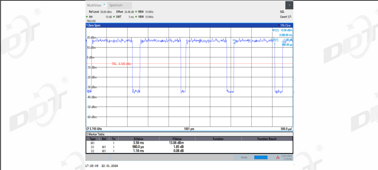
11N20MIMO_Ant2_5745
