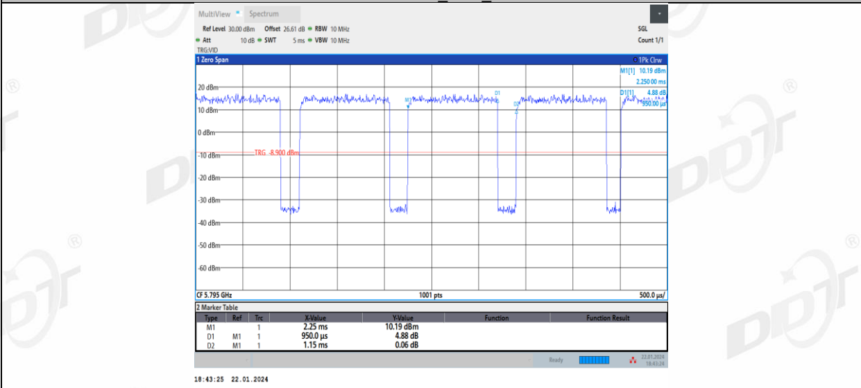
11AC40MIMO_Ant2_5795
