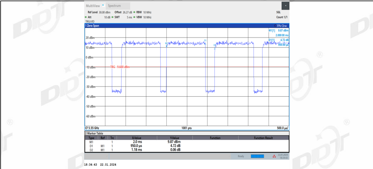
11AC40MIMO_Ant2_5550
