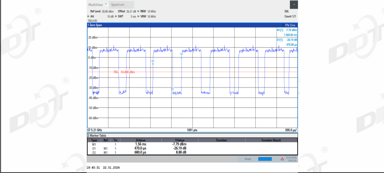
11AC80MIMO_Ant2_5210
