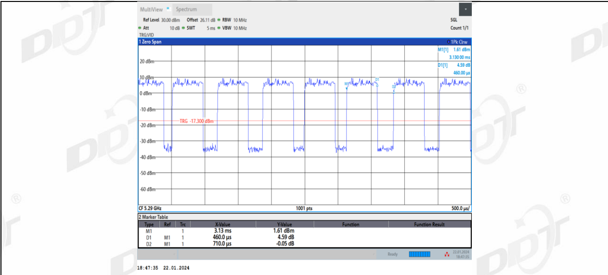
11AC80MIMO_Ant2_5290
