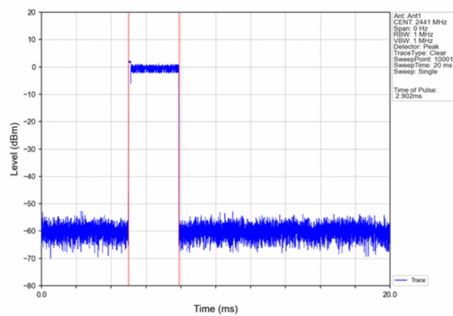
Pi/4DQPSK_2DH5_HOPP_Ant1_NTNV
