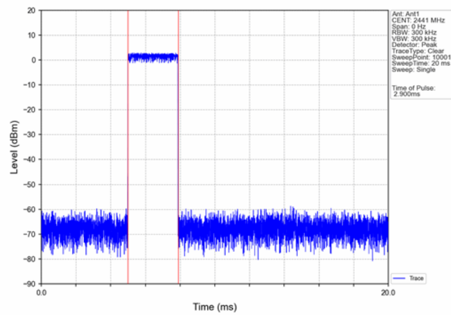
GFSK_DH5_HOPP_Ant1_NTNV
