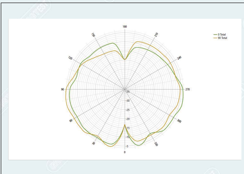
Phi=0°&amp; Phi=90°_2500 MHz
