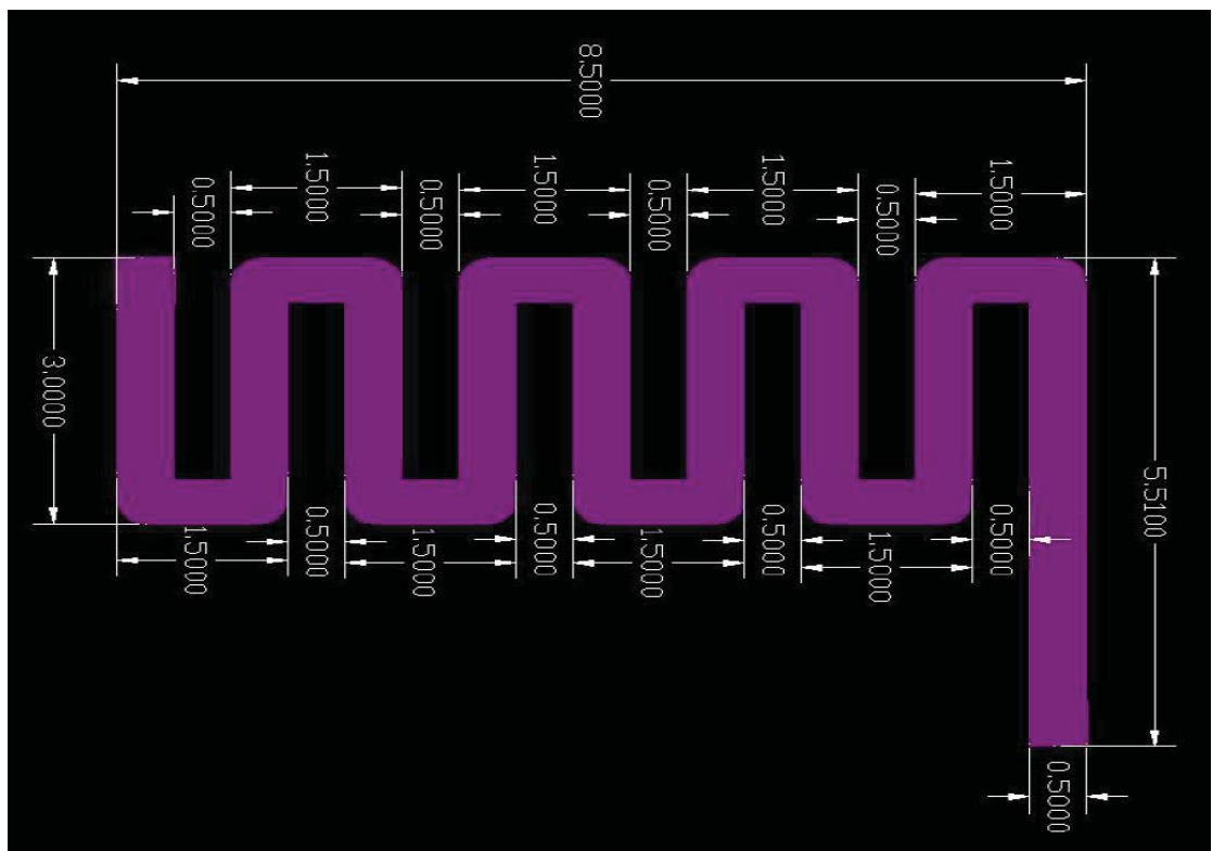
天线尺寸
