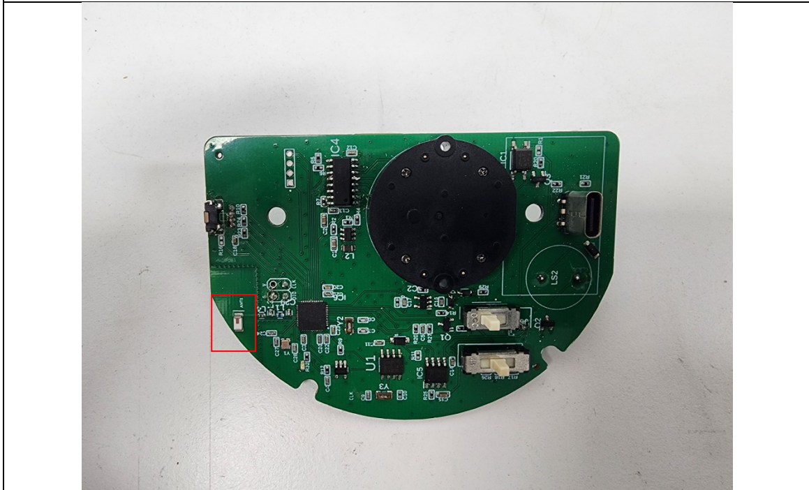
ANTENNA(2.4 GHz)
