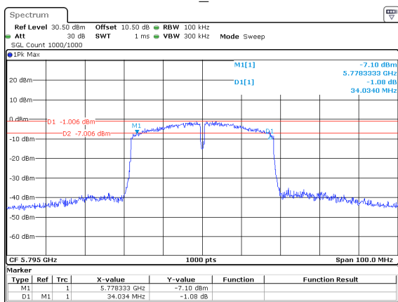
802.11n40_5795MHz
