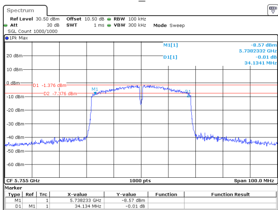
802.11n40_5755MHz
