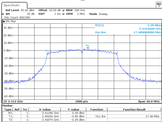
802.11n20_2412MHz
