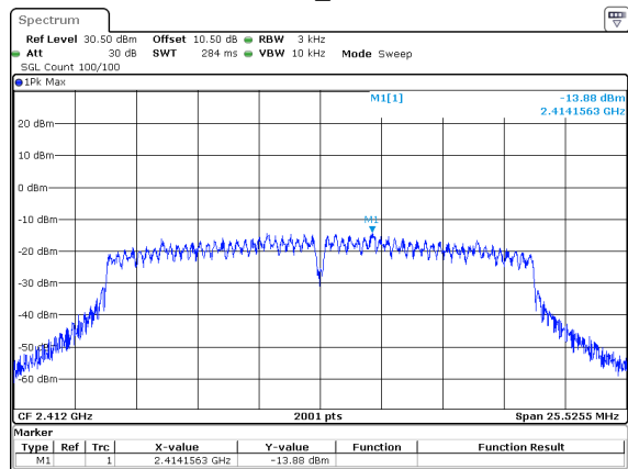
802.11n20_2412MHz
