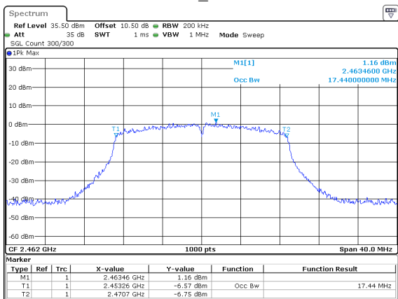
802.11n20_2462MHz
