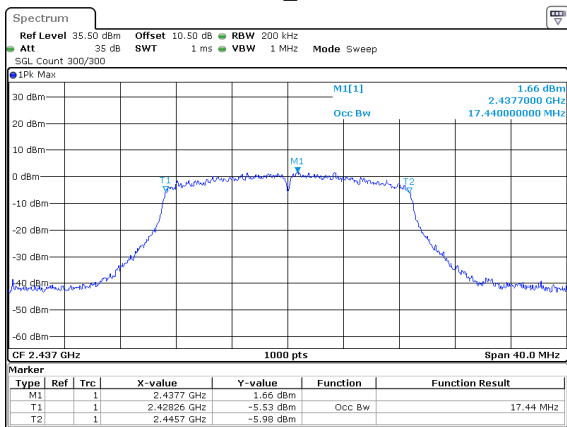
802.11n20_2437MHz
