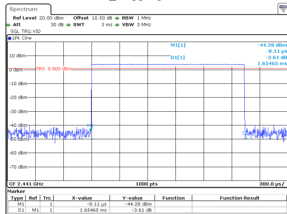
DH3_Hopping 1.655ms
