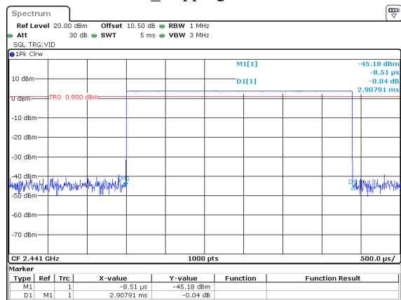
DH5_Hopping 2.908ms
