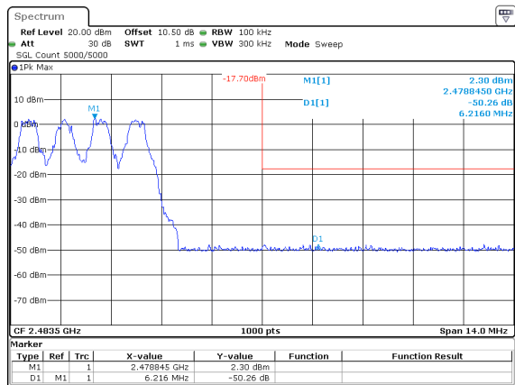
DH1_Hopping_Upper
