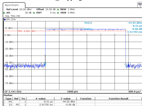
2DH5_Hopping 2.918ms
