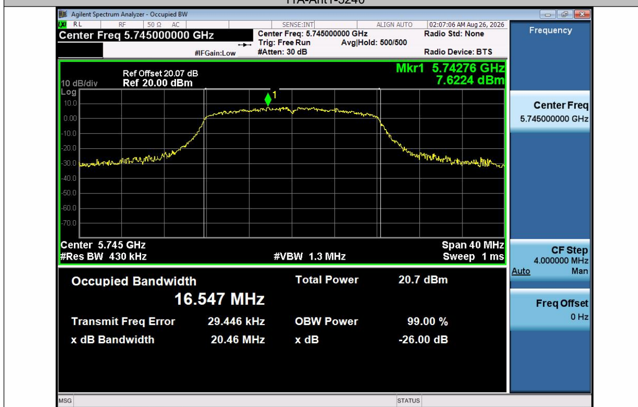
11A-Ant1-5745
