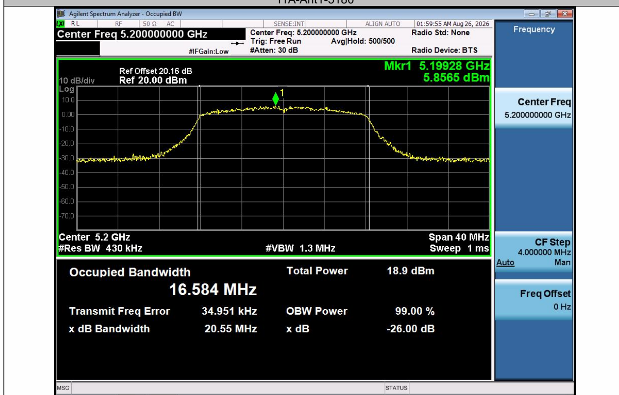
11A-Ant1-5200
