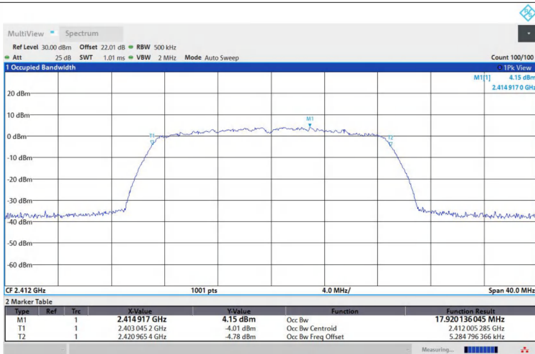
11N20MIMO-Ant1-2412
