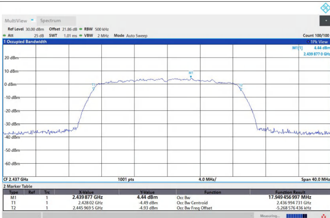
11N20MIMO-Ant1-2437
