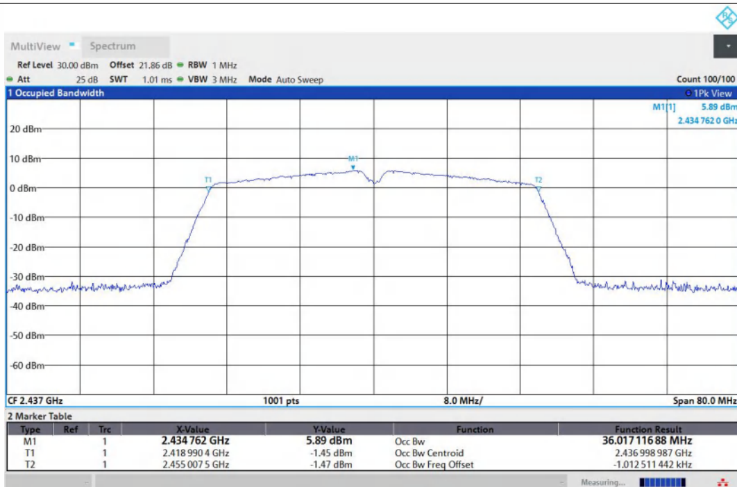
11N40MIMO-Ant1-2437
