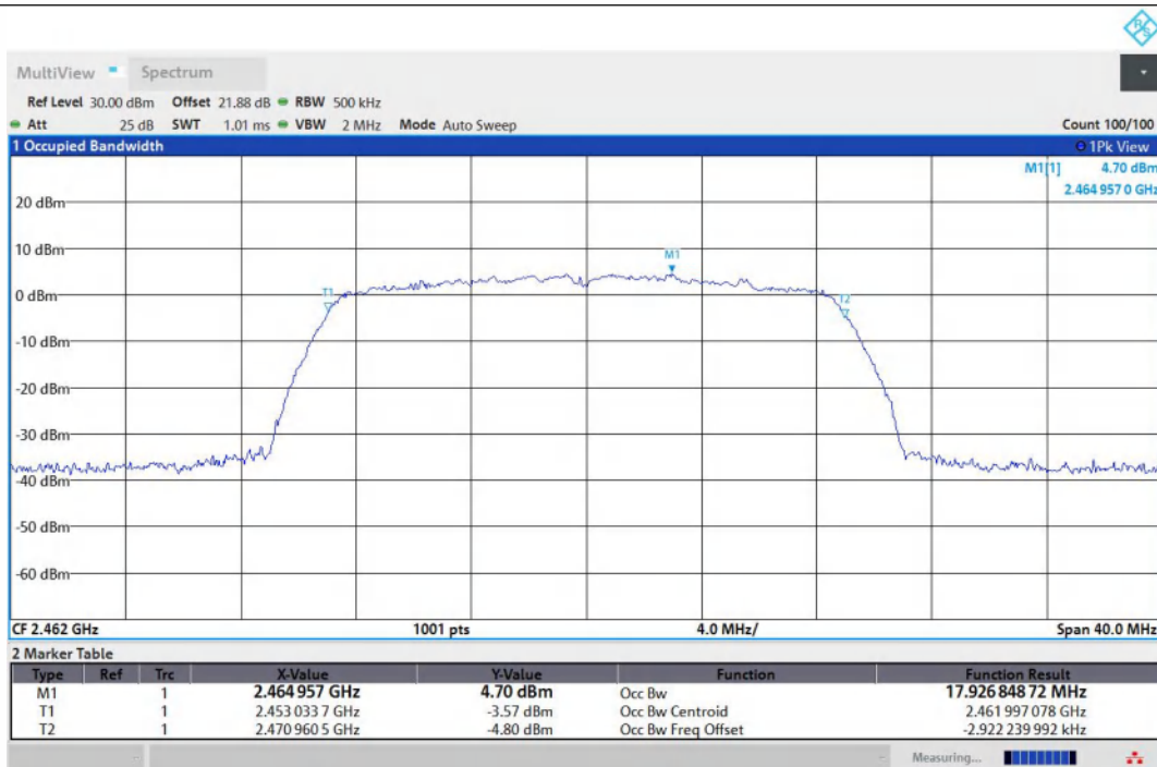
11N20MIMO-Ant1-2462
