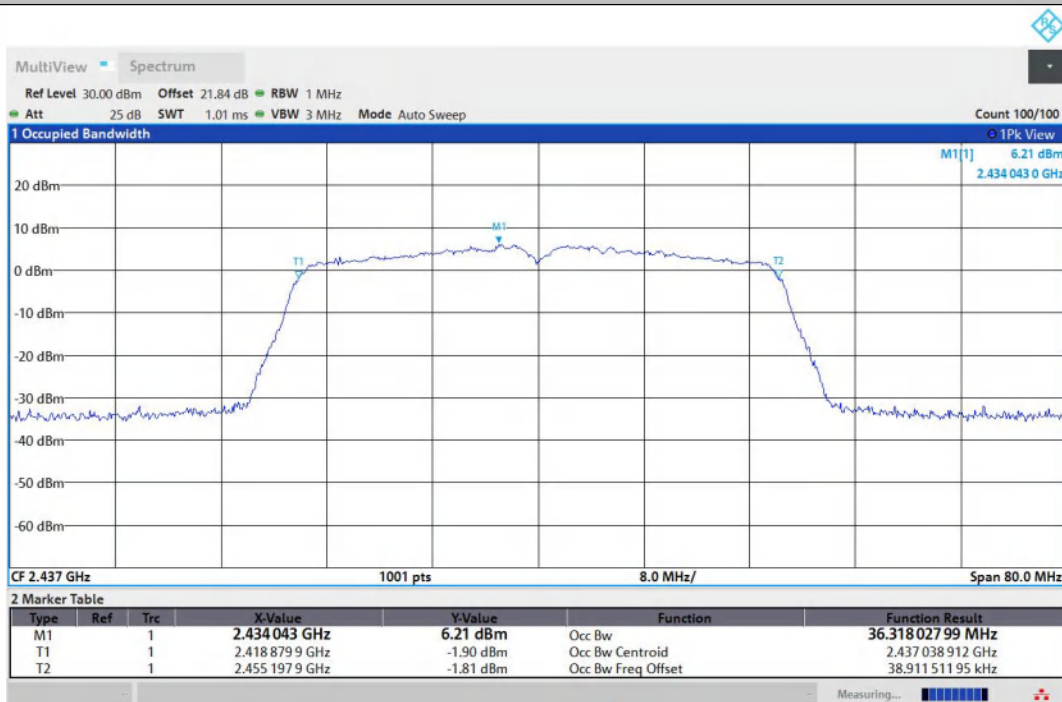
11N40MIMO-Ant2-2437
