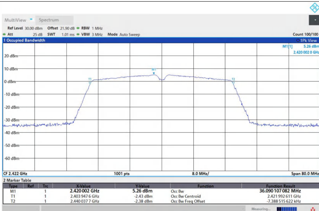
11N40MIMO-Ant1-2422
