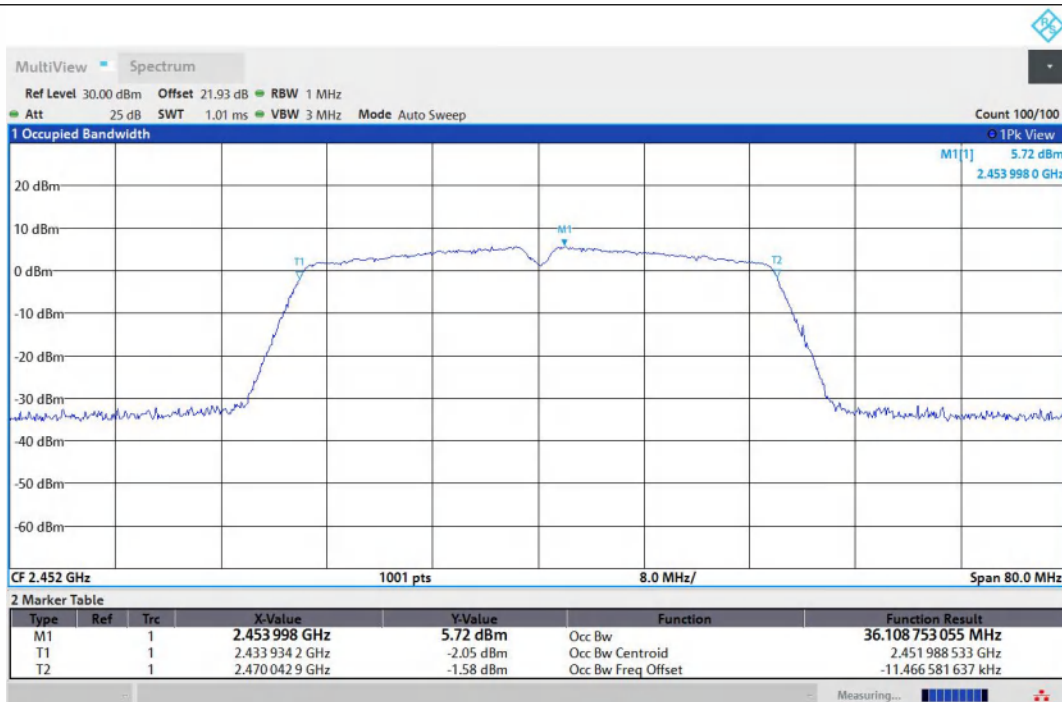
11N40MIMO-Ant1-2452
