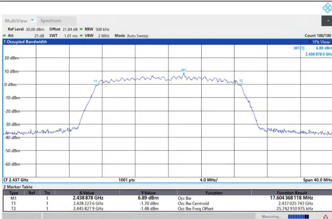
11N20MIMO-Ant2-2437
