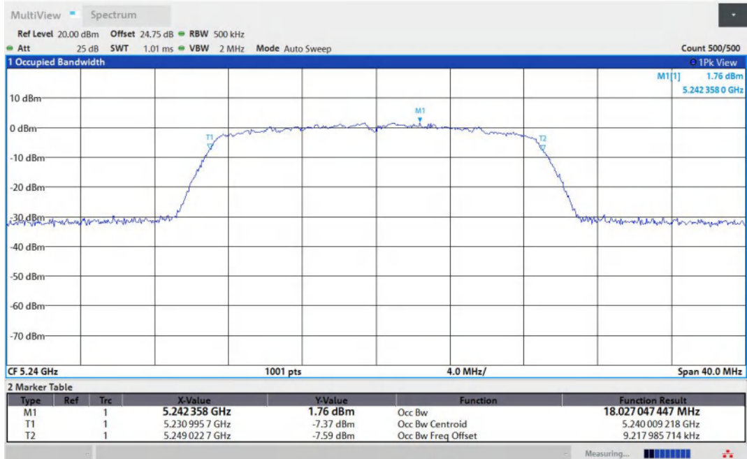
11N20MIMO-Ant1-5240
