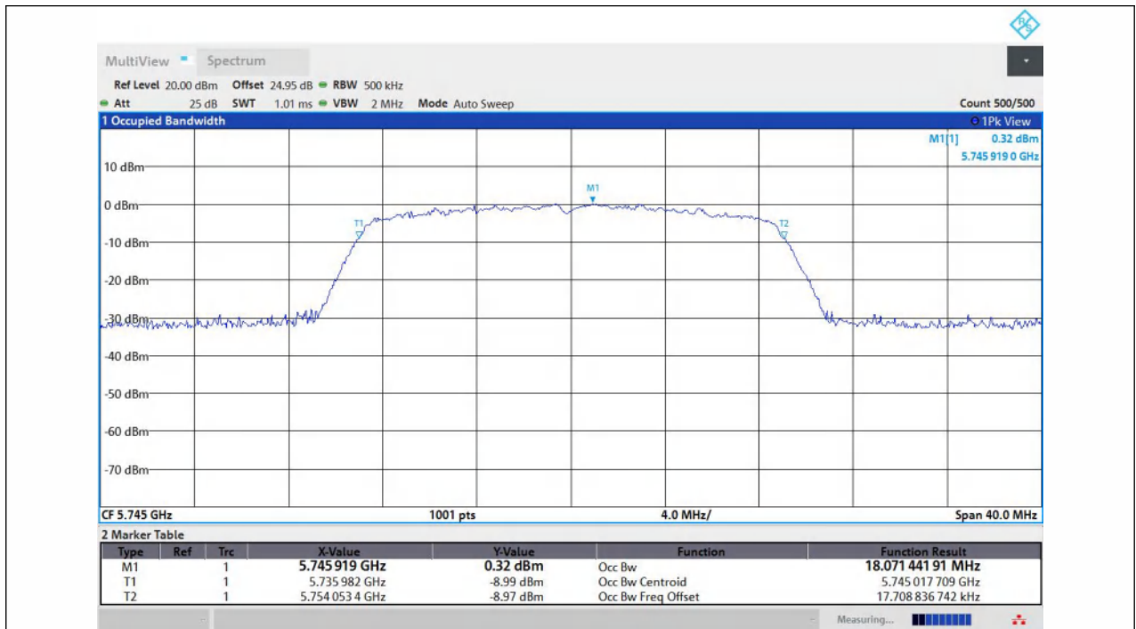
11N20MIMO-Ant1-5745
