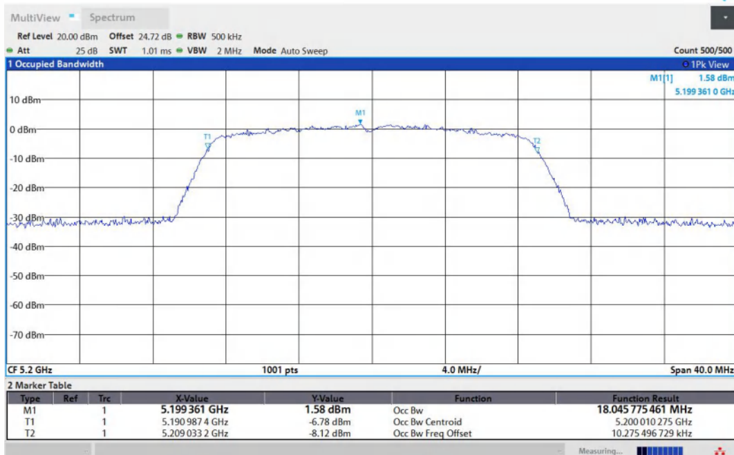
11AC20MIMO-Ant1-5200
