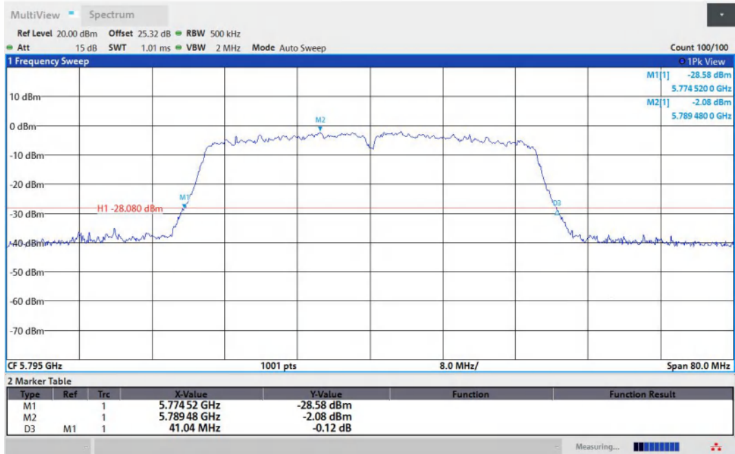
11N40MIMO-Ant1-5795
