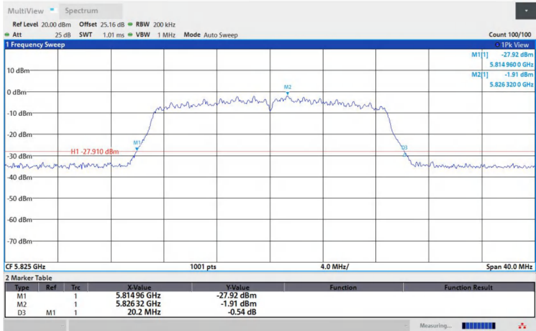
11N20MIMO-Ant1-5825
