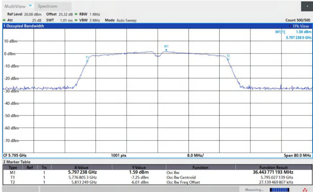
11N40MIMO-Ant1-5795
