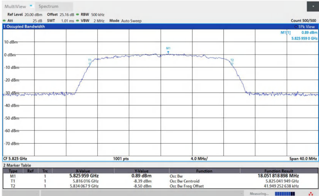
11N20MIMO-Ant1-5825
