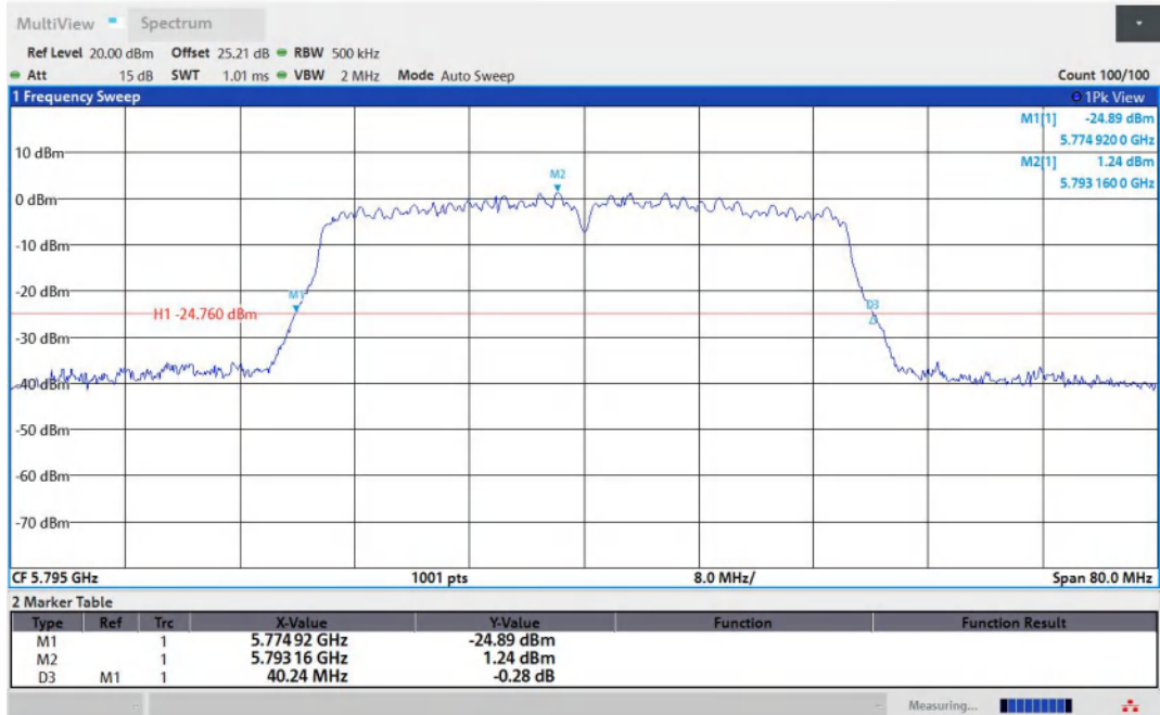
11N40MIMO-Ant2-5795
