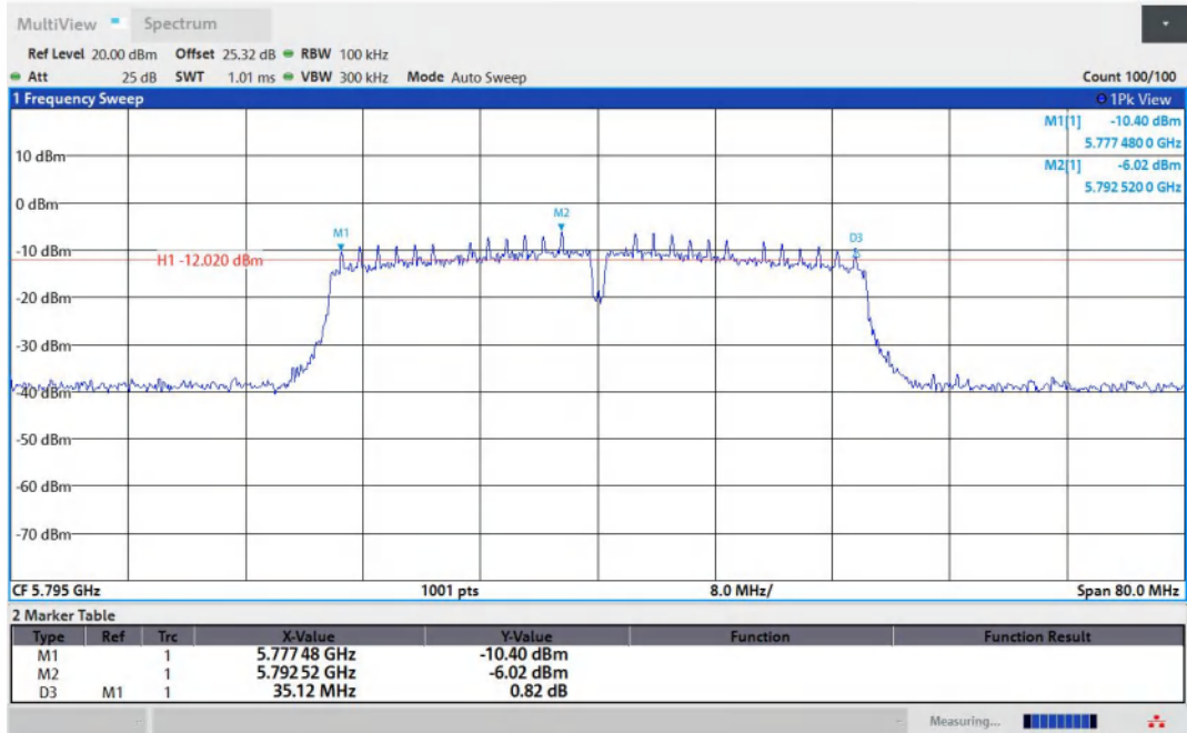
11N40MIMO-Ant1-5795-PASS
