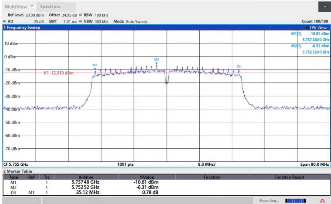
11N40MIMO-Ant1-5755-PASS
