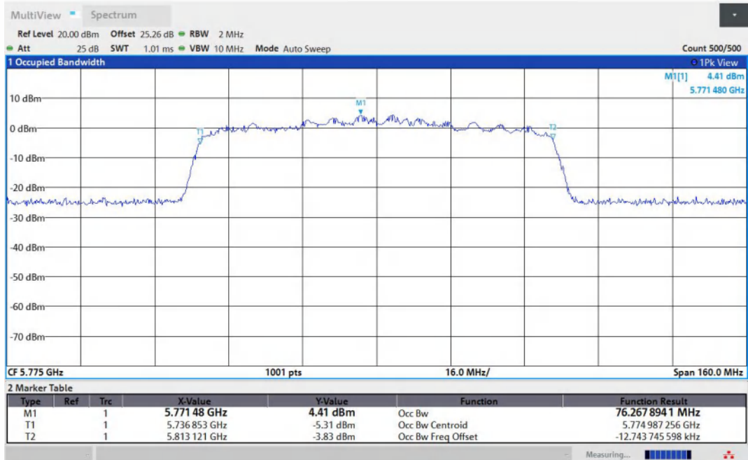
11AC80MIMO-Ant1-5775
