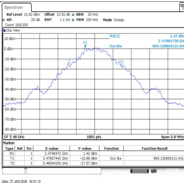
DH5-Ant1-2480
