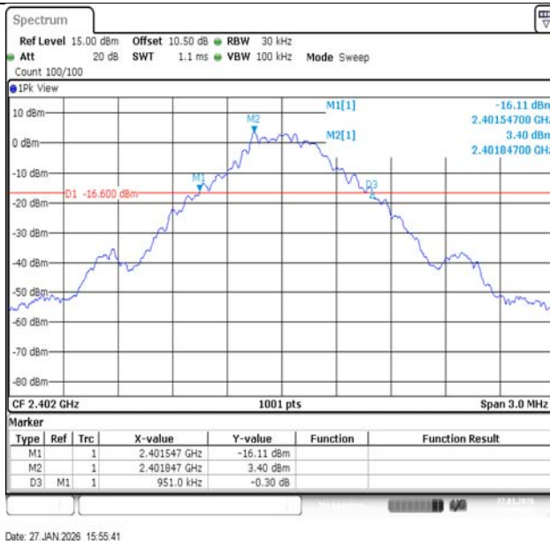
DH5-Ant1-2402
