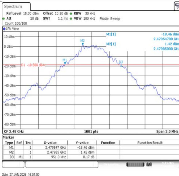
DH5-Ant1-2480
