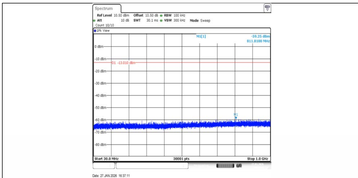
BLE_2M-Ant1-2402-30~1000-PASS
