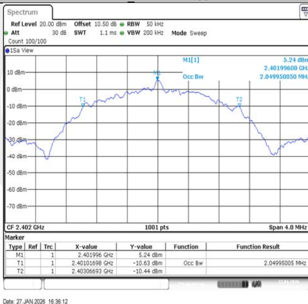
BLE_2M-Ant1-2402
