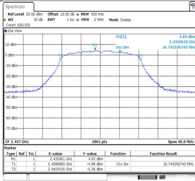
11G-Ant1-2437
