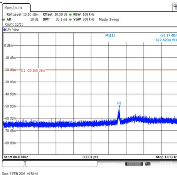
11G-Ant1-2437-30~1000-PASS
