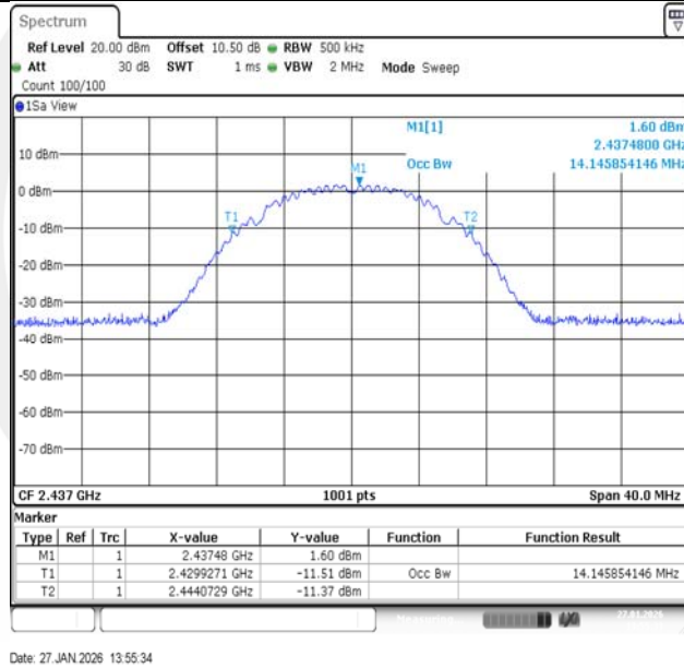
11B-Ant1-2437
