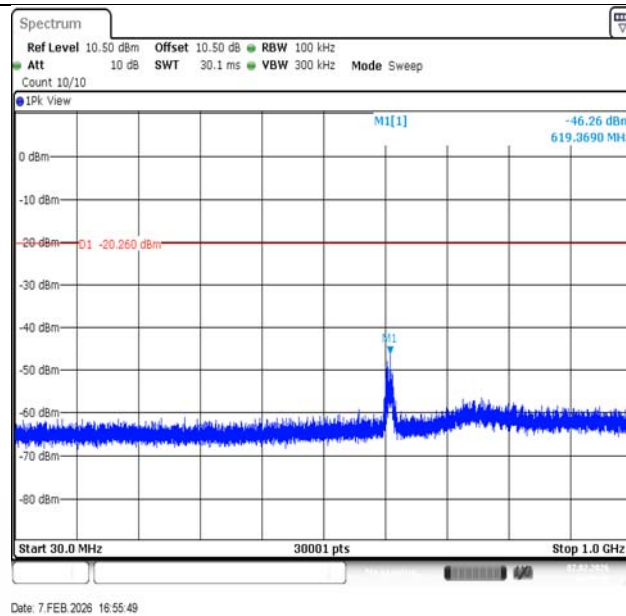
11G-Ant1-2412-30~1000-PASS
