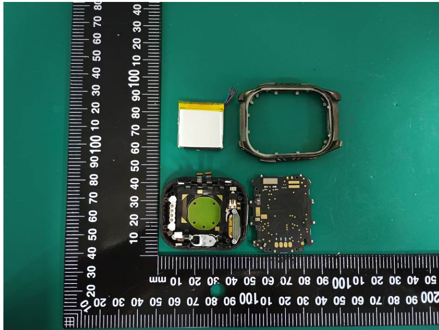
BT&BLE ANT
