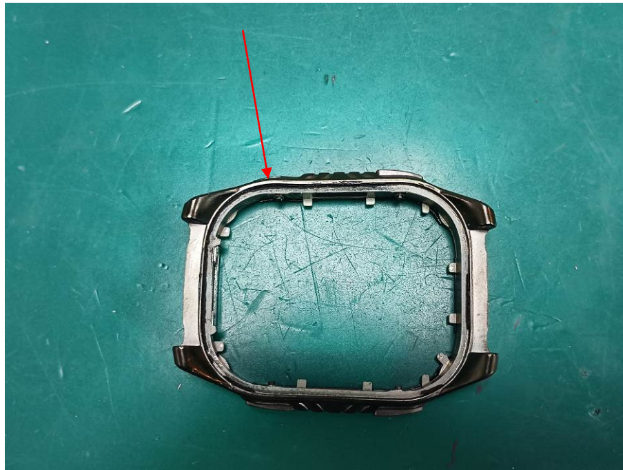
BT&BLE ANT
