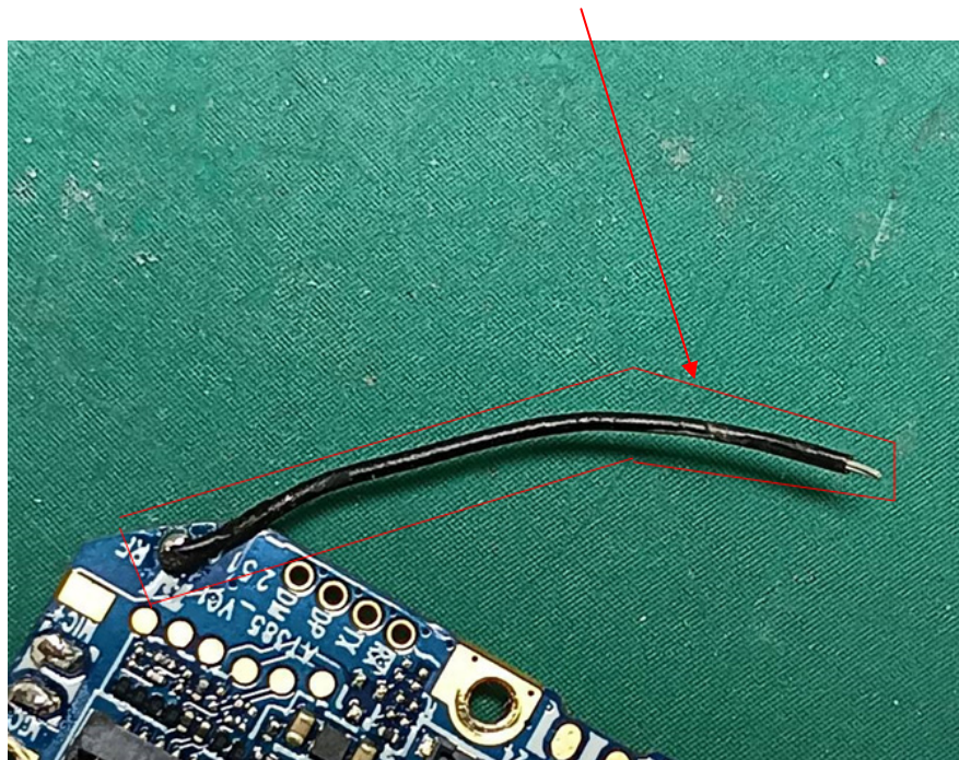
Antenna
