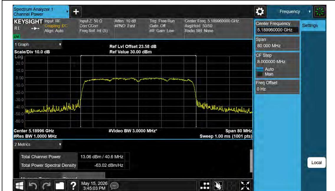
11AX40MIMO-Ant0-5230-PASS
