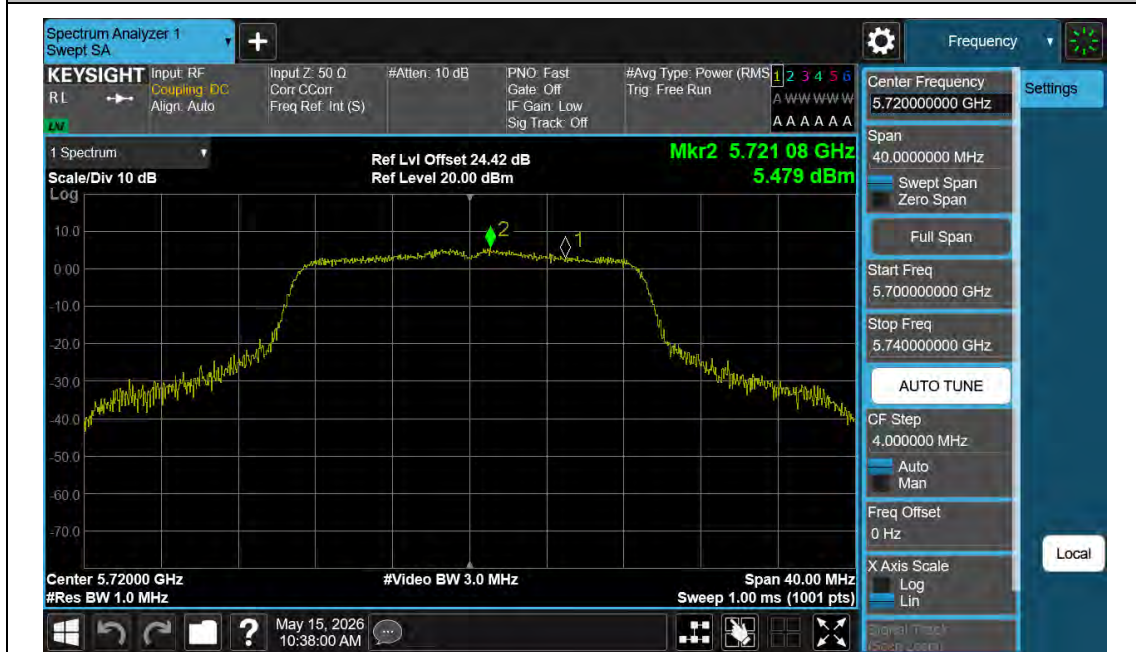
11N20MIMO-Ant0-5720_UNII-3-PASS
