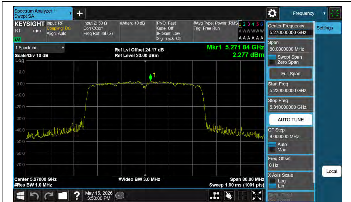
11AX40MIMO-Ant1-5270-PASS
