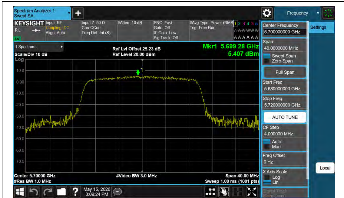
11AX20MIMO-Ant1-5700-PASS
