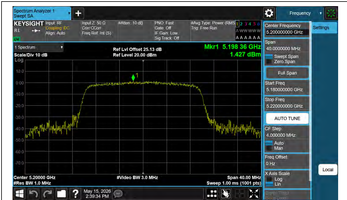
11AX20MIMO-Ant1-5200-PASS
