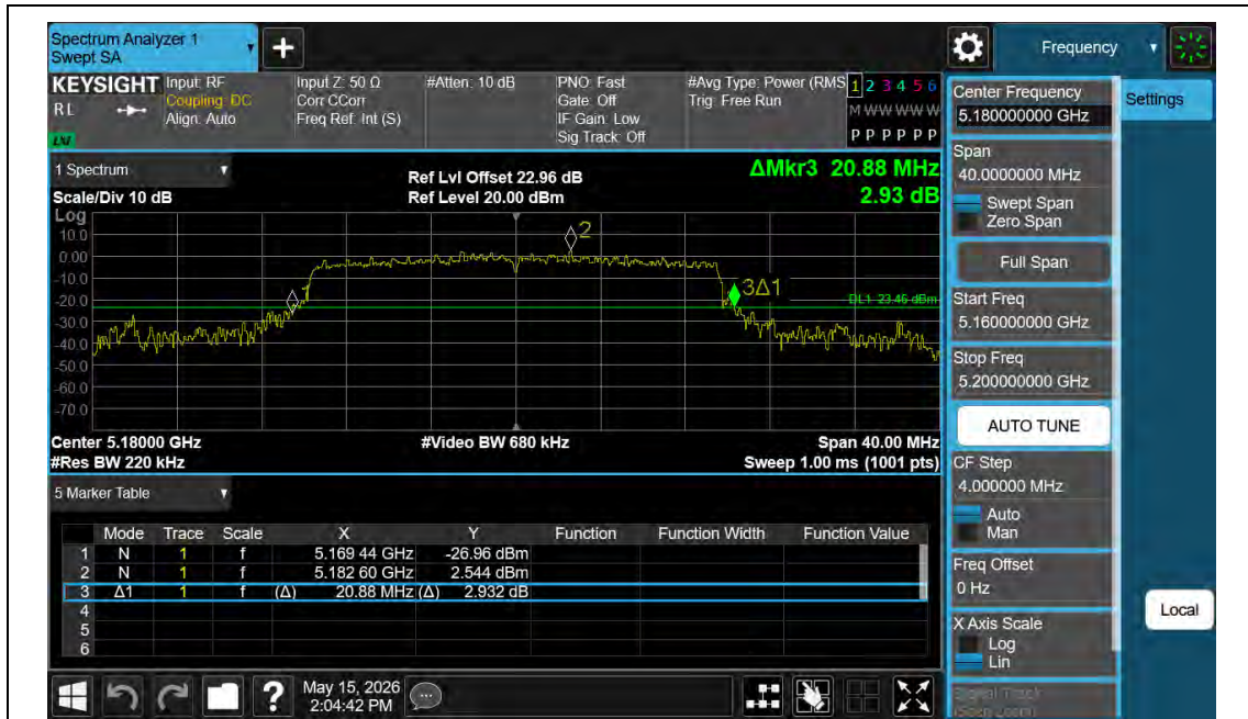
11AX20MIMO-Ant1-5180
