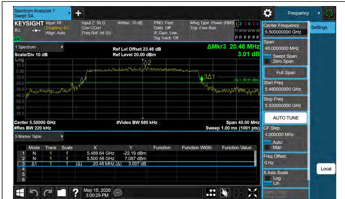
11AX20MIMO-Ant1-5500
