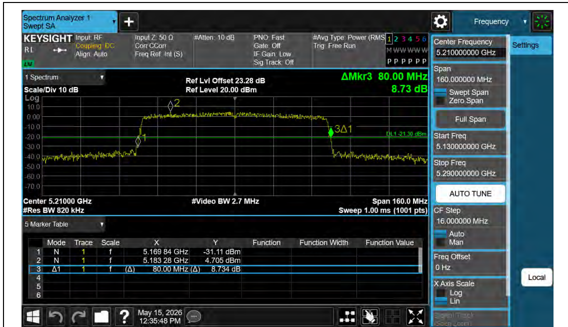
11AC80MIMO-Ant1-5210
