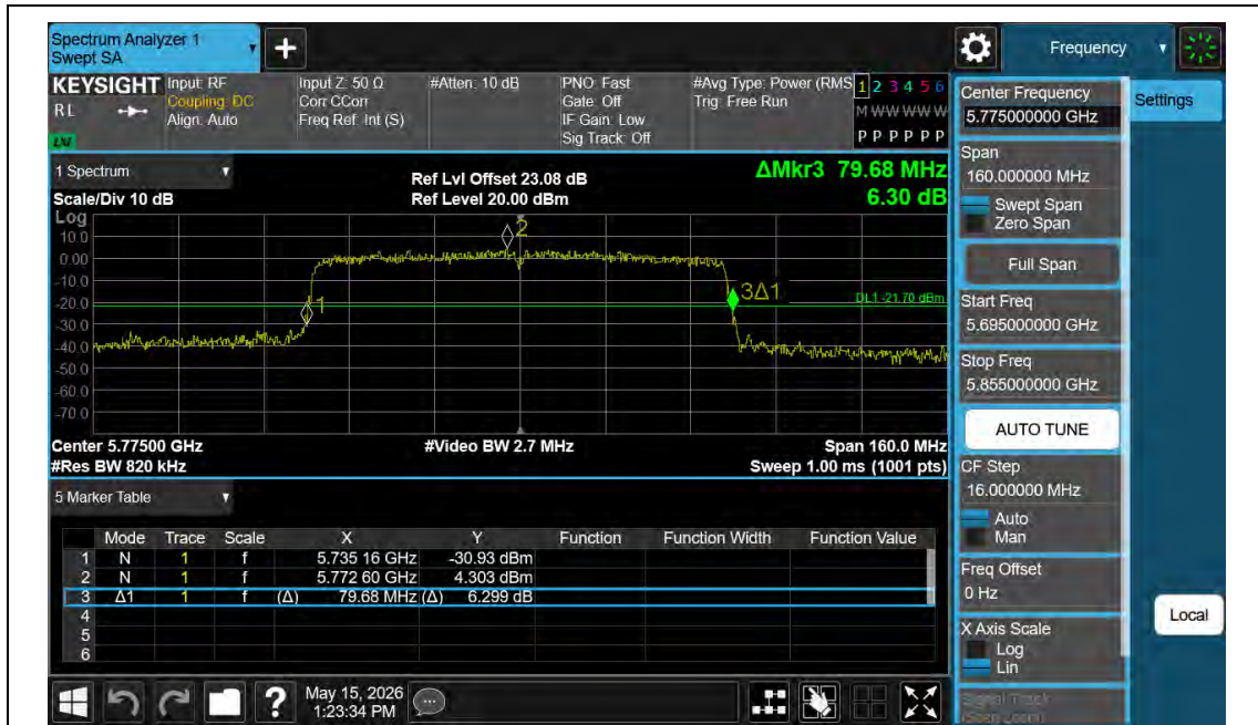
11AC80MIMO-Ant1-5775
