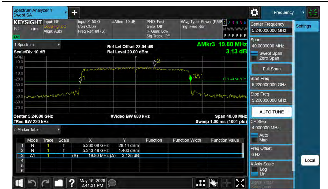
11AX20MIMO-Ant1-5240
