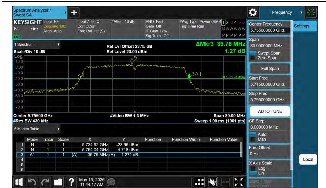
11AC40MIMO-Ant1-5755
