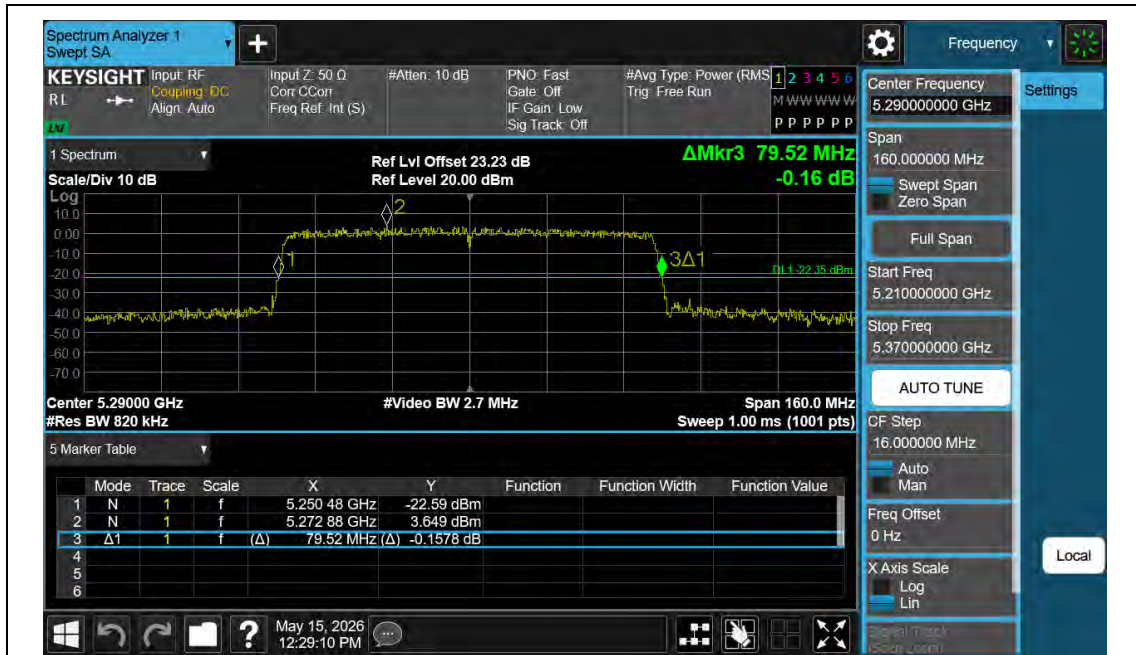
11AC80MIMO-Ant1-5290
