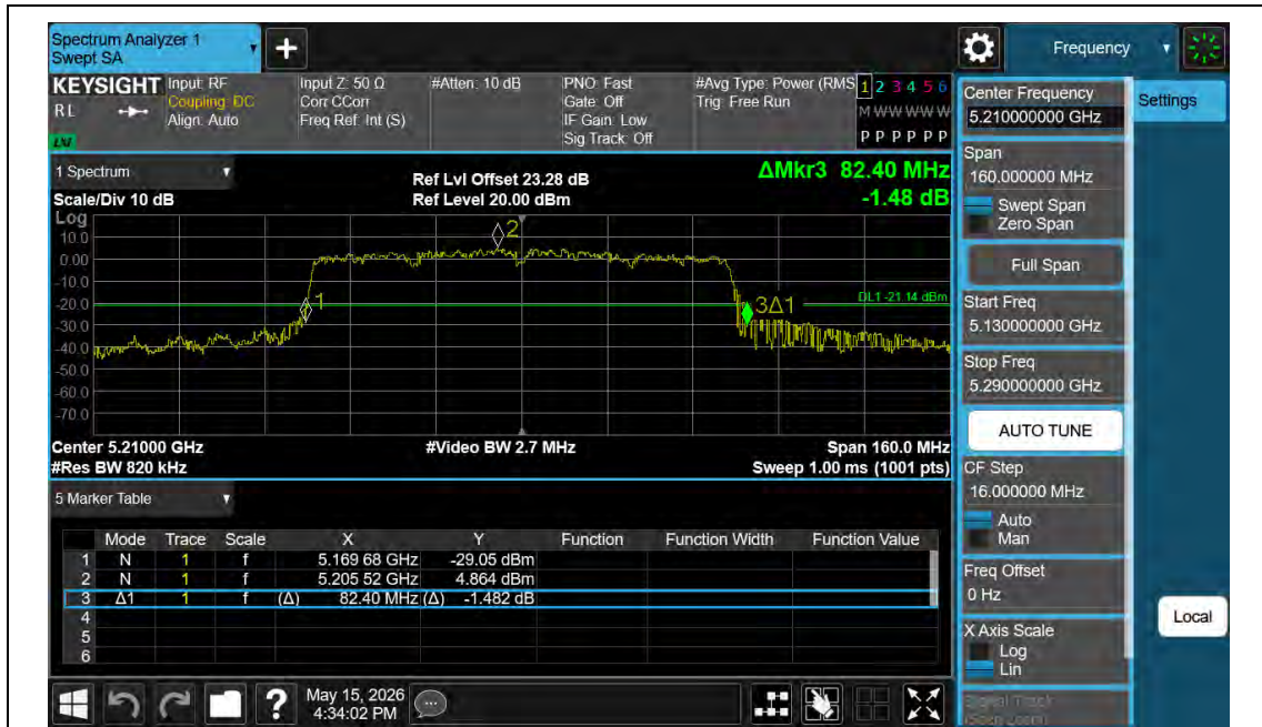
11AX80MIMO-Ant1-5210
