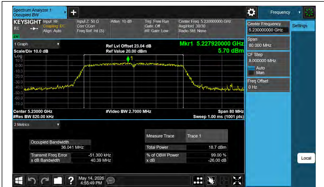
11N40MIMO-Ant1-5230
