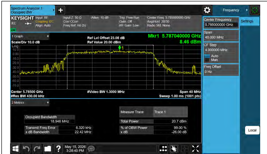
11AX20MIMO-Ant1-5785
