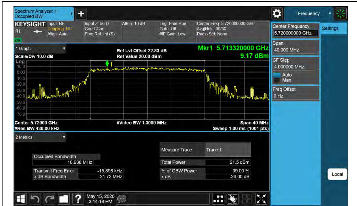
11AX20MIMO-Ant1-5720
