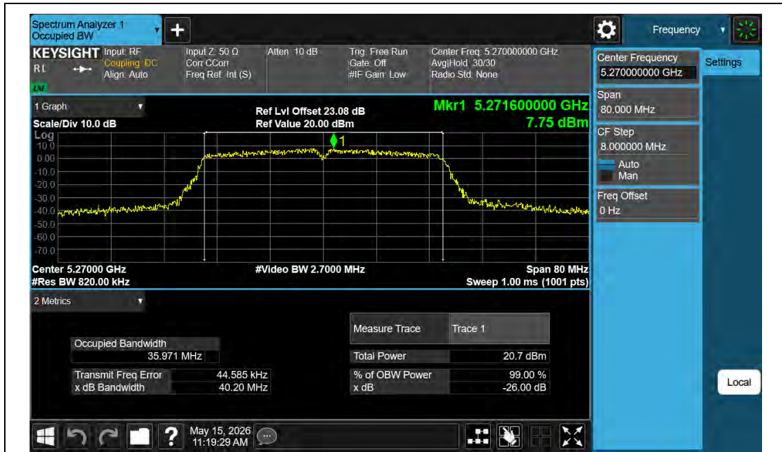
11AC40MIMO-Ant1-5270
