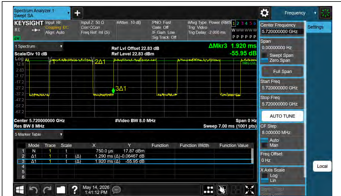
NTNV-11N20MIMO-Ant1-5720
