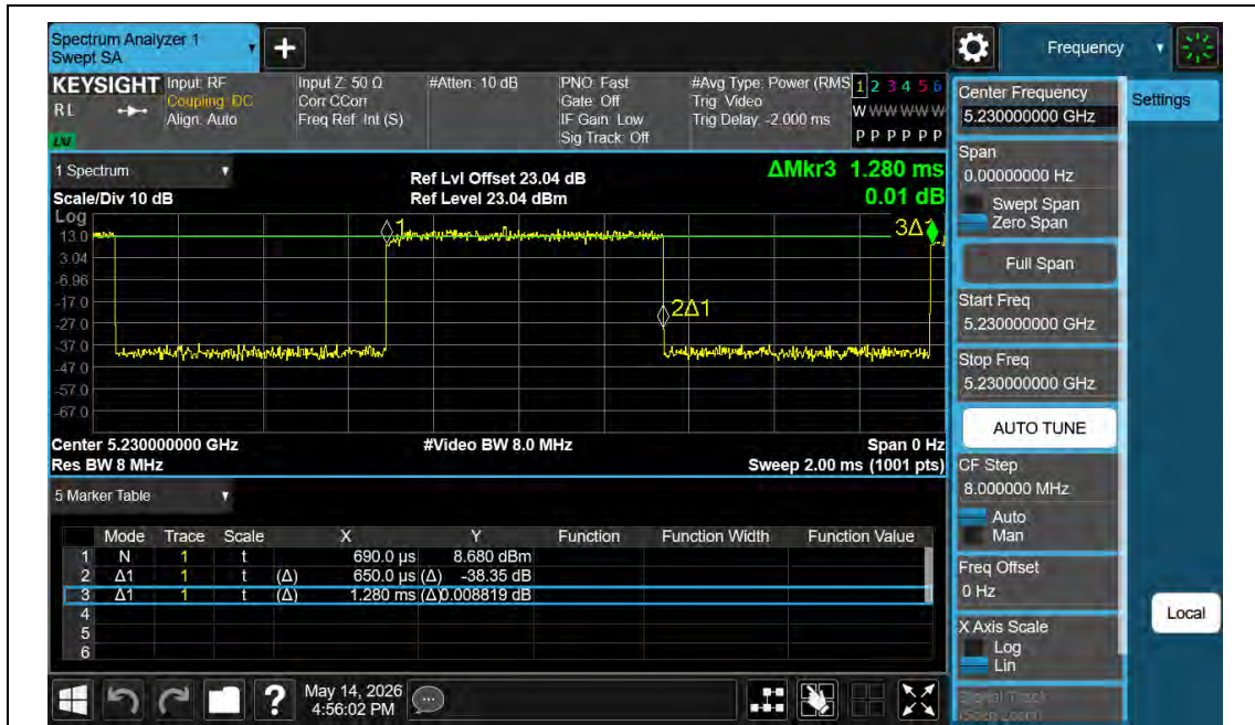
NTNV-11N40MIMO-Ant1-5230
