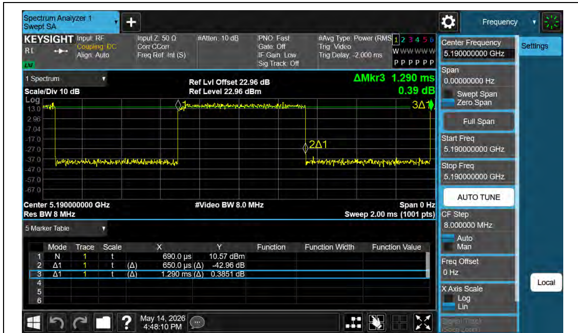
NTNV-11N40MIMO-Ant1-5190
