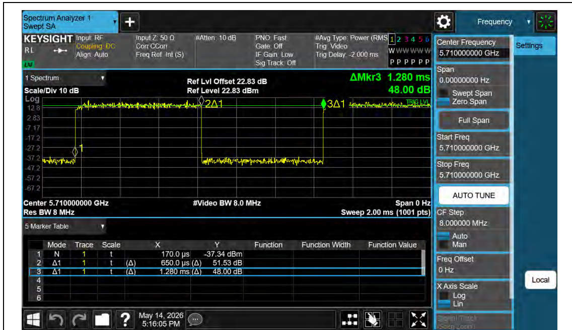
NTNV-11N40MIMO-Ant1-5710
