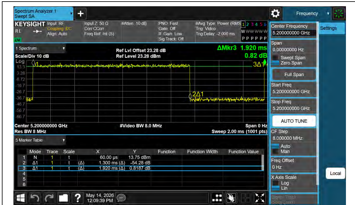
NTNV-11N20MIMO-Ant1-5200
