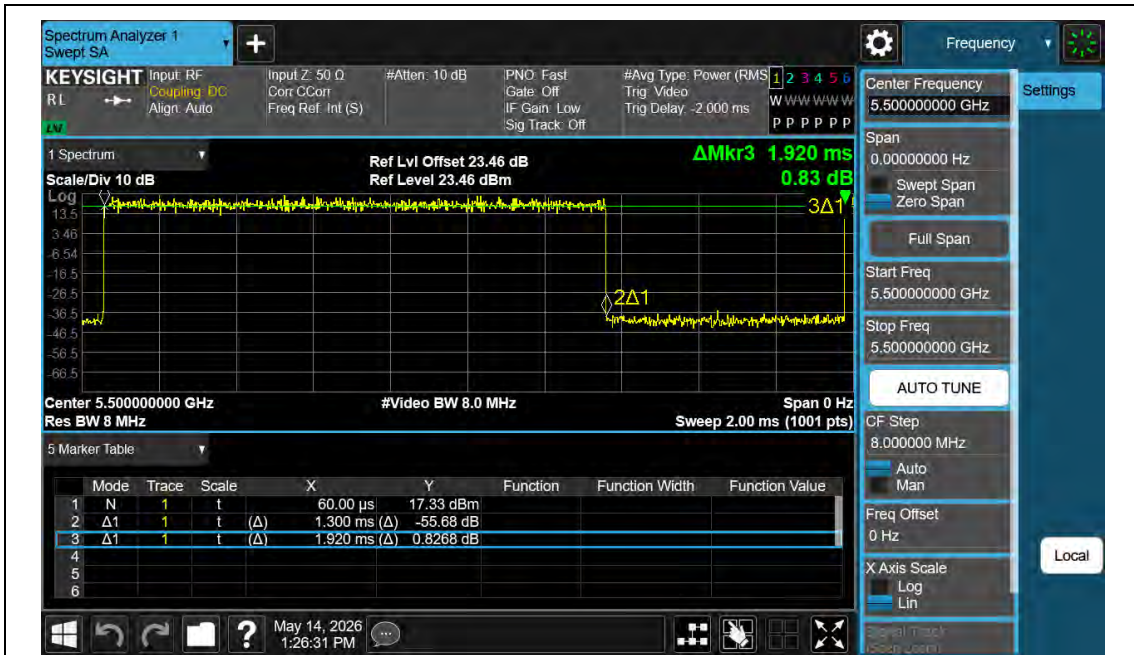
NTNV-11N20MIMO-Ant1-5500
