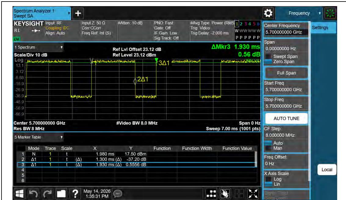
NTNV-11N20MIMO-Ant1-5700
