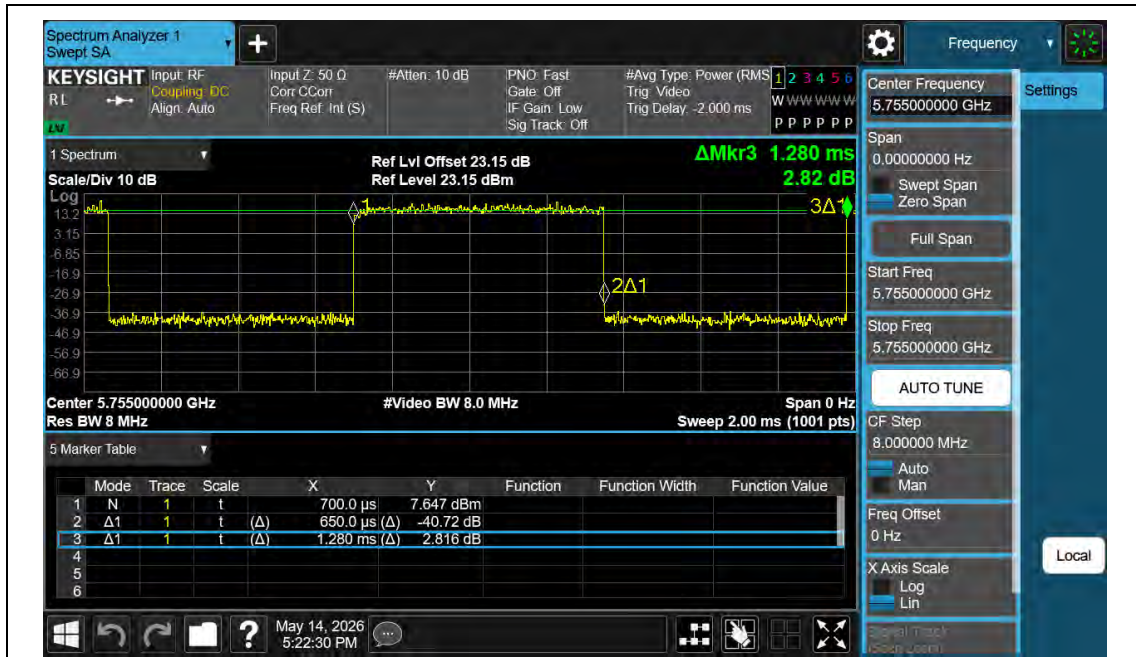
NTNV-11N40MIMO-Ant1-5755
