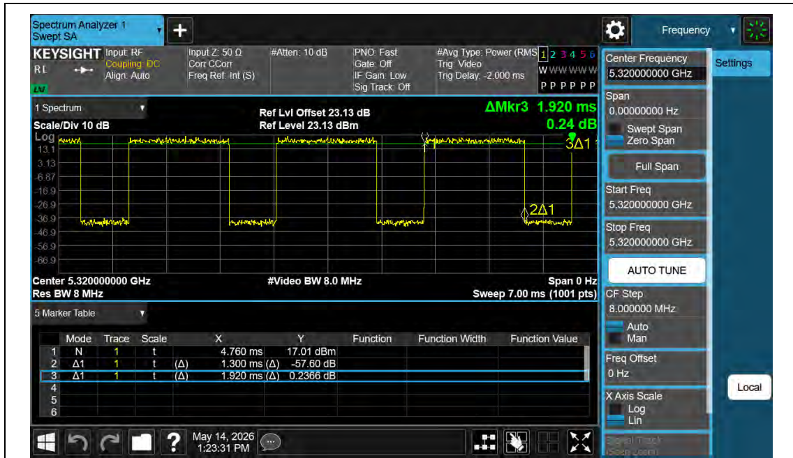
NTNV-11N20MIMO-Ant1-5320
