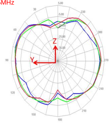
E2 Face 5745MHz
