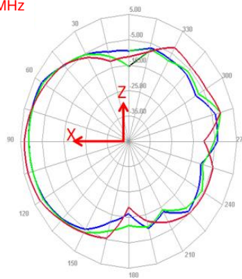
E1 Face 5745MHz
